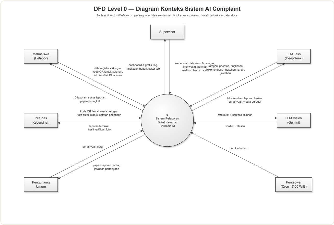
Gambar 1. DFD Level 0: seluruh sistem sebagai satu proses, dikelilingi tujuh entitas eksternal.
