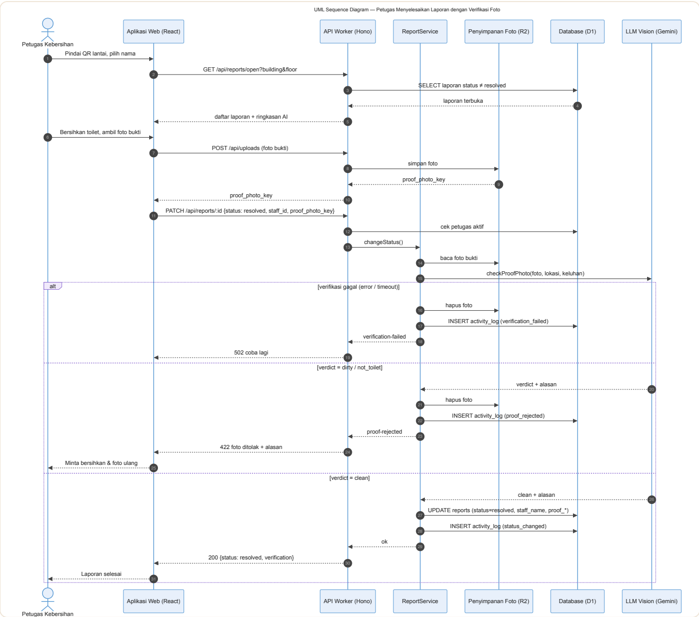
Gambar 15. Urutan kejadian saat petugas menyelesaikan laporan dengan foto bukti.
