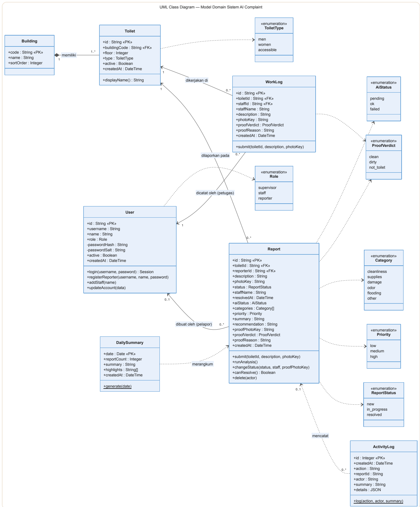
Gambar 13. Class diagram: tujuh kelas data dan tujuh daftar nilai tetap (enumeration).
