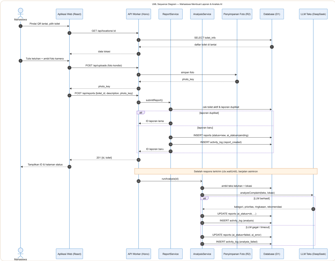
Gambar 14. Urutan kejadian saat mahasiswa membuat laporan, sampai AI selesai menganalisisnya.
