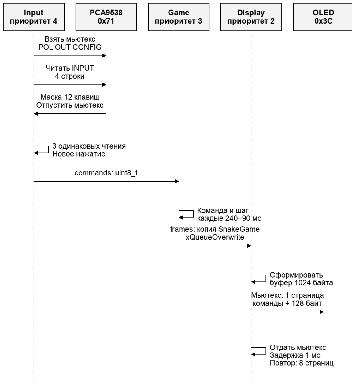
Рисунок 2 — Опрос клавиатуры передача команд и обновление OLED
