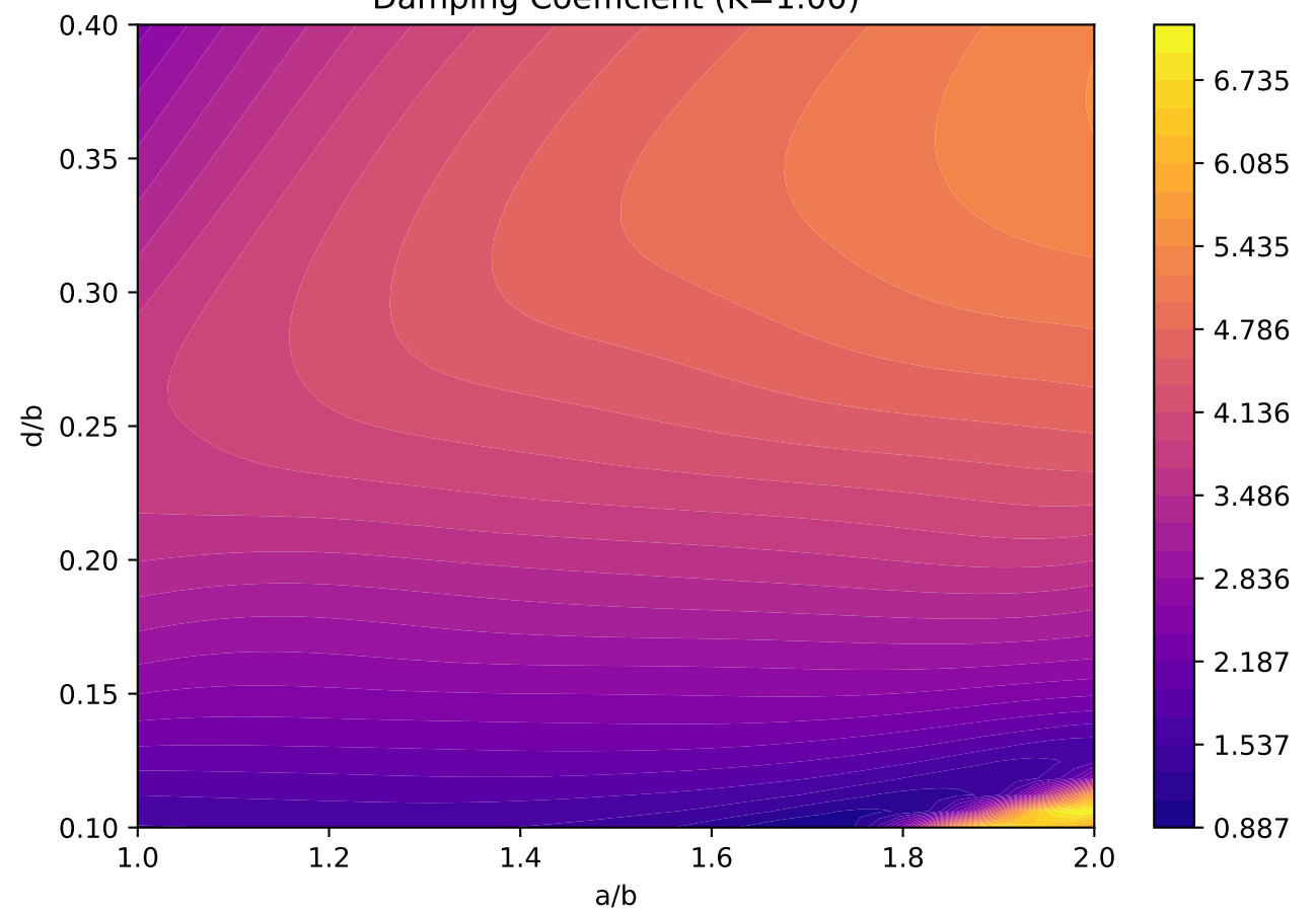
Damping Coefficient (K=1.00)
