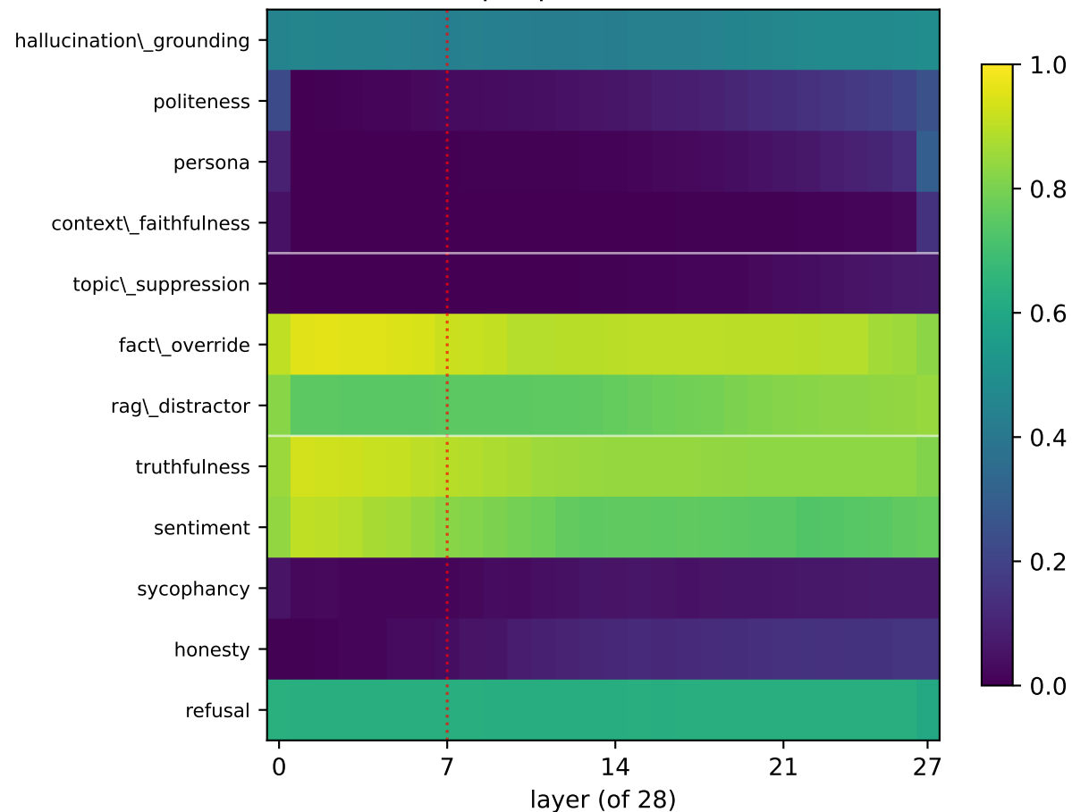
per-pair variance
