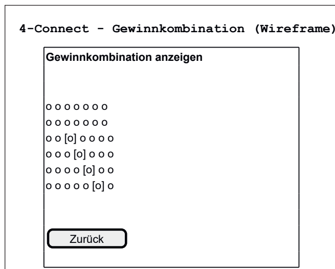
Abbildung: Wireframe – Gewinnkombination anzeigen
