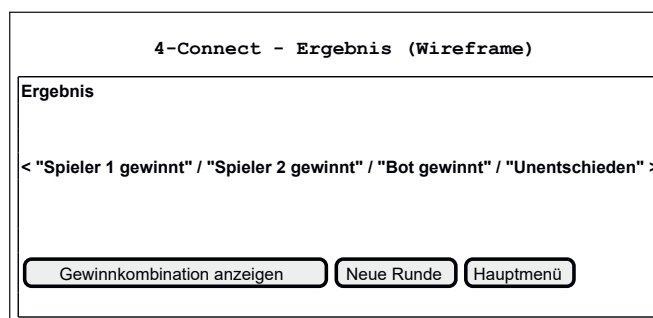
Abbildung: Wireframe – Ergebnisbildschirm
