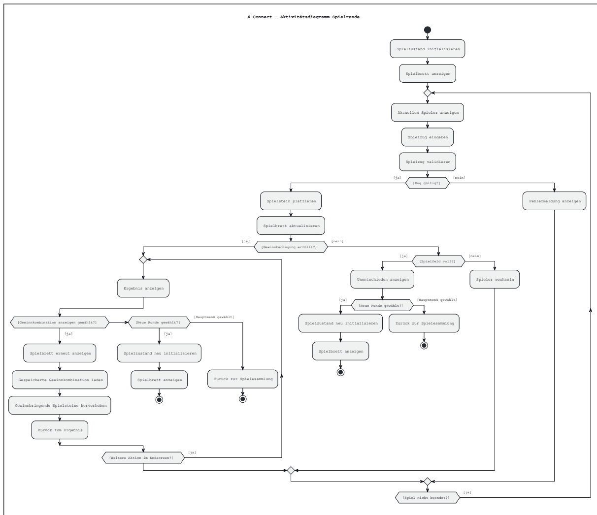
Abbildung: Aktivitätsdiagramm – Spielrunde
