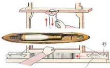
飛び杼のしくみ。杼は縦糸の間に経糸を通す装置。右手でひもを引けば、杼が右端のように左右を往復する。
