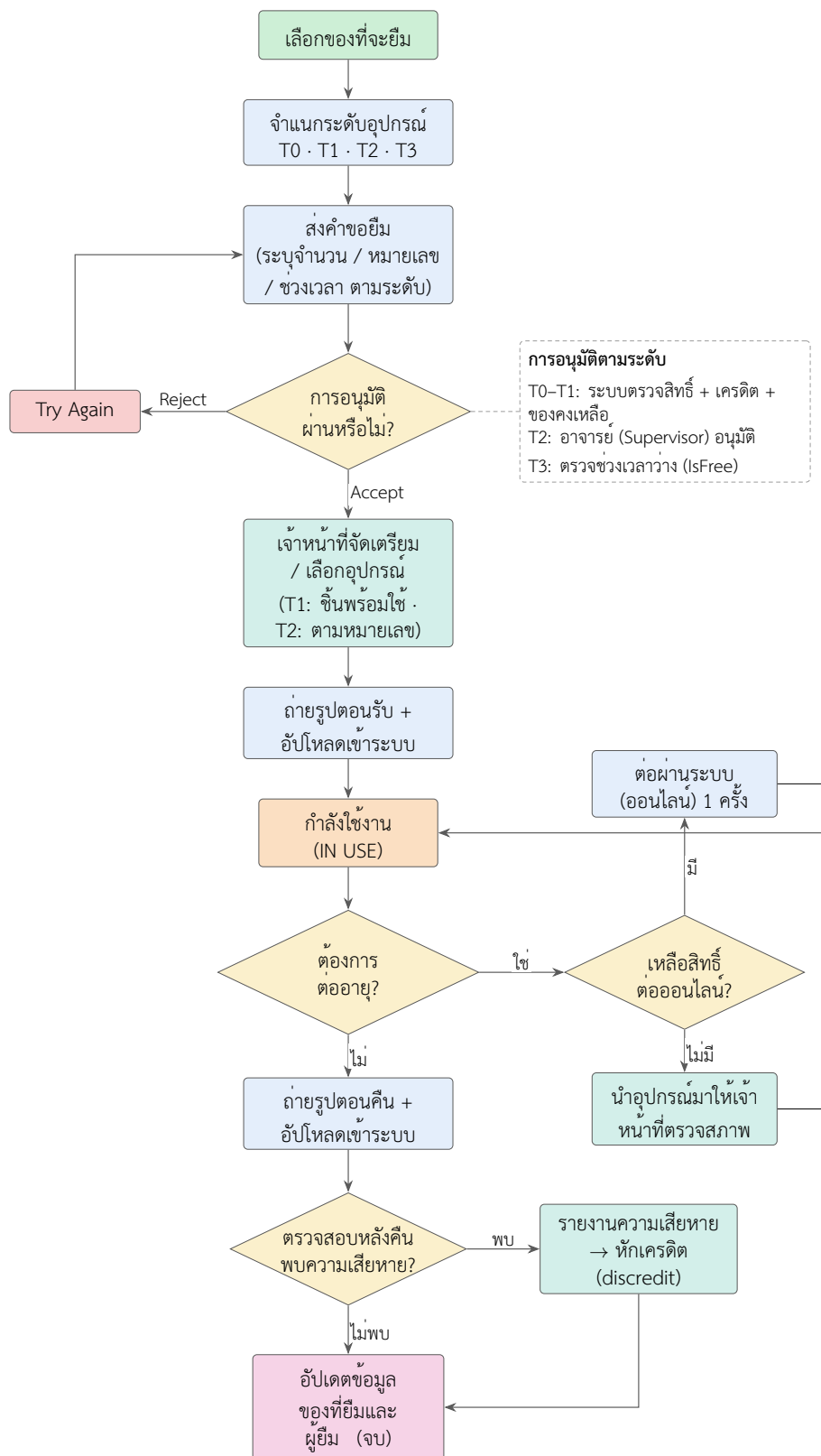
รูปที่ 2: ผังงานกระบวนการยืม-คืนอุปกรณ์ รหัสสี: สีฟ้า = ขั้นตอนของผู้ยืม, สีเขียวอมฟ้า = ขั้นตอนของเจ้าหน้าที่ (Staff), สีเหลือง = จุดตัดสินใจ, สีส้ม = ระหว่างใช้งาน, สีชมพู = อัปเดตข้อมูลเมื่อจบรายการ
