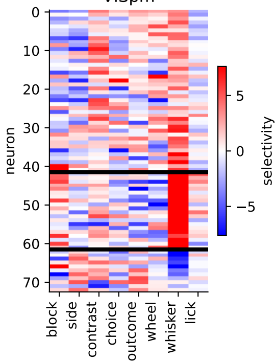
null data
