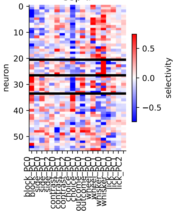
null data
