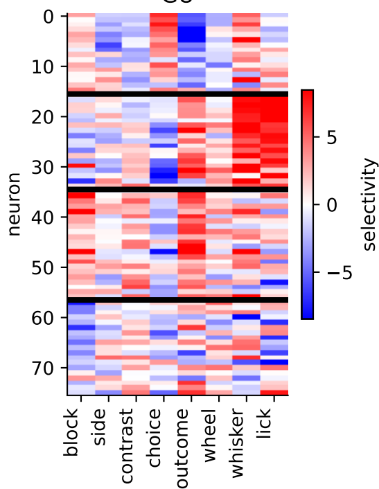
null data
