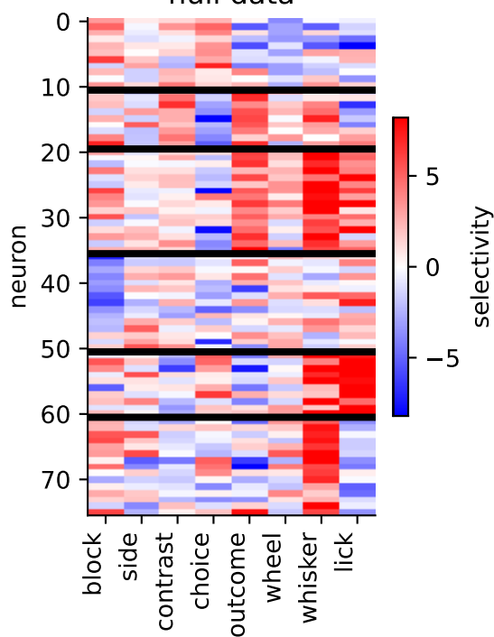
ss_z: 0.07
