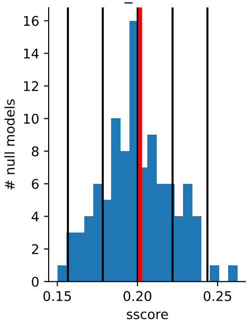
ss_z: 0.07
