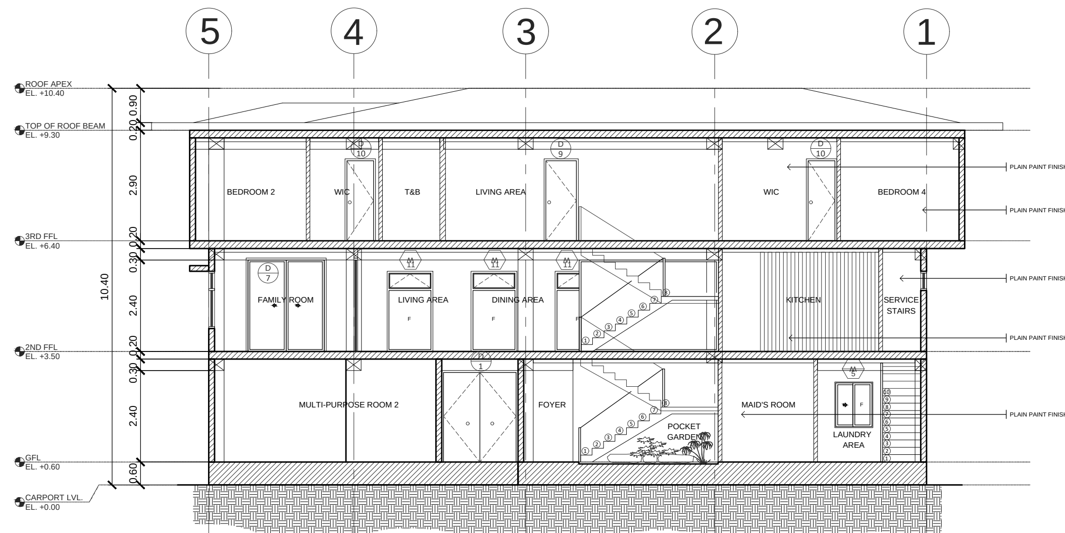
ARANETA RESIDENCE 2 LONGITUDINAL SECTION A-06 SCALE: 1:100 MTS
