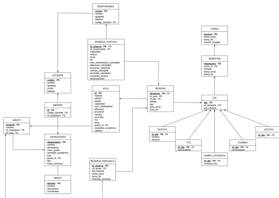
Figura C.2: Modelo relacional
