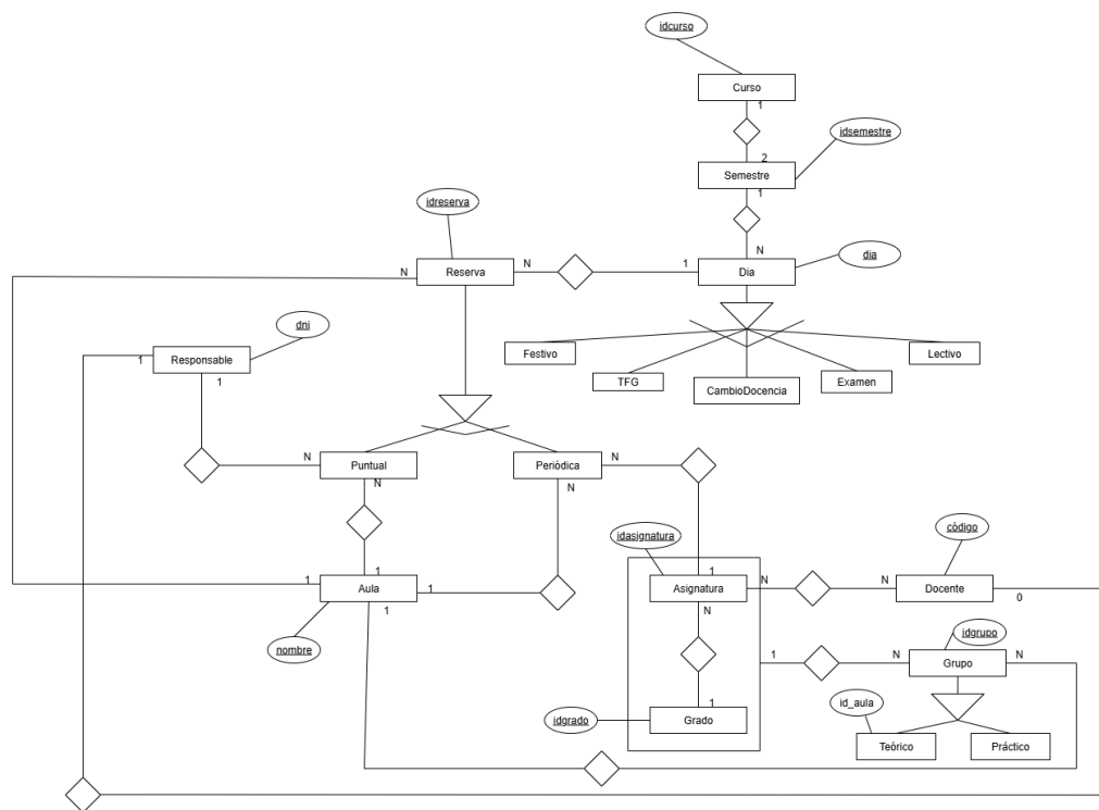
Figura C.1: Diagrama entidad-relación
