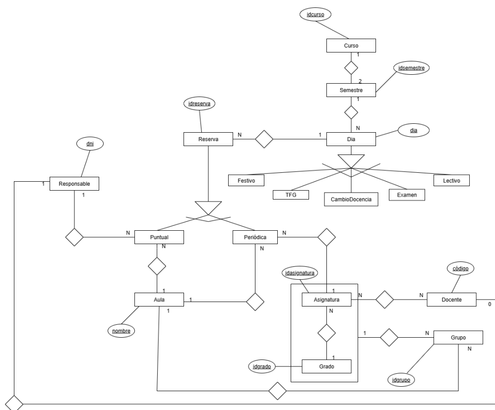
Figura C.1: Diagrama entidad-relación
