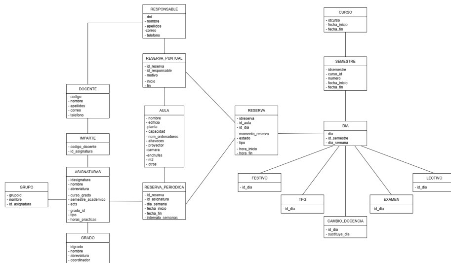
Figura C.2: Modelo relacional
