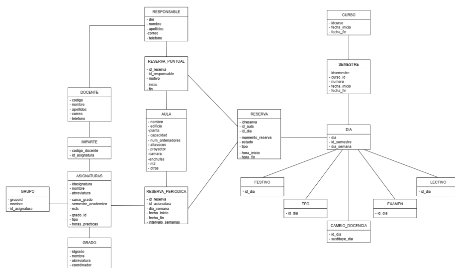
Figura C.2: Modelo relacional
