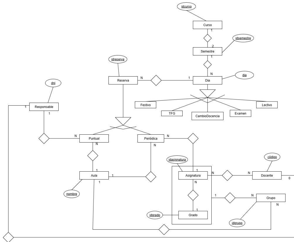
Figura C.1: Diagrama entidad-relación
