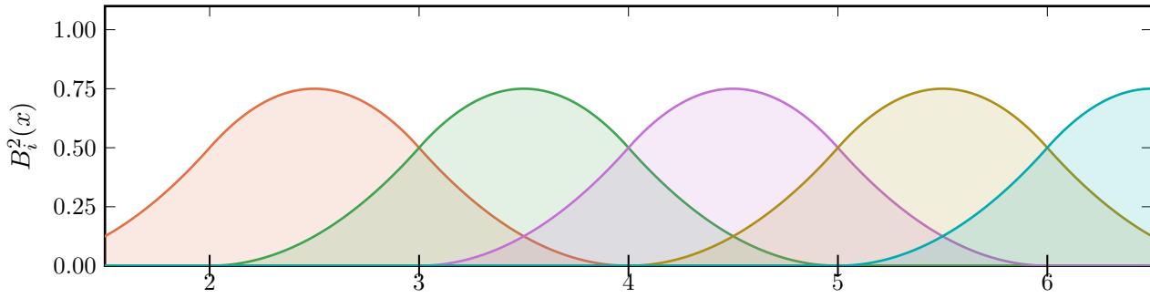
c) Grado p = 2 (Cuadrático)
