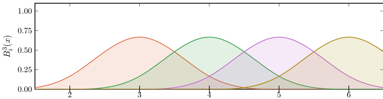
d) Grado p = 3 (Cúbico)
