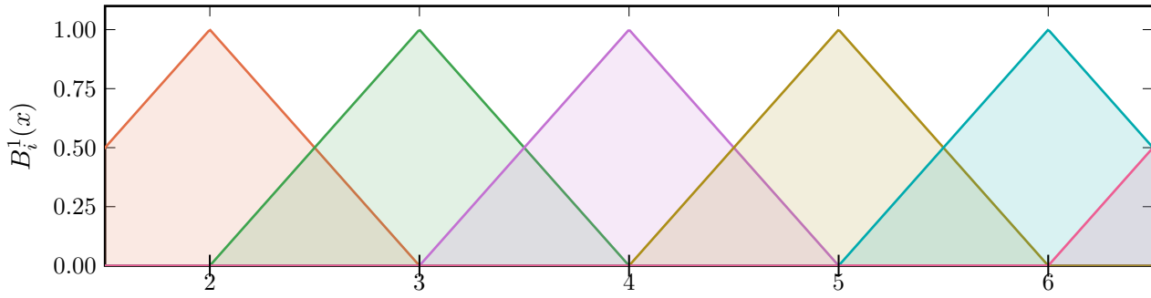
b) Grado p = 1 (Lineal)
