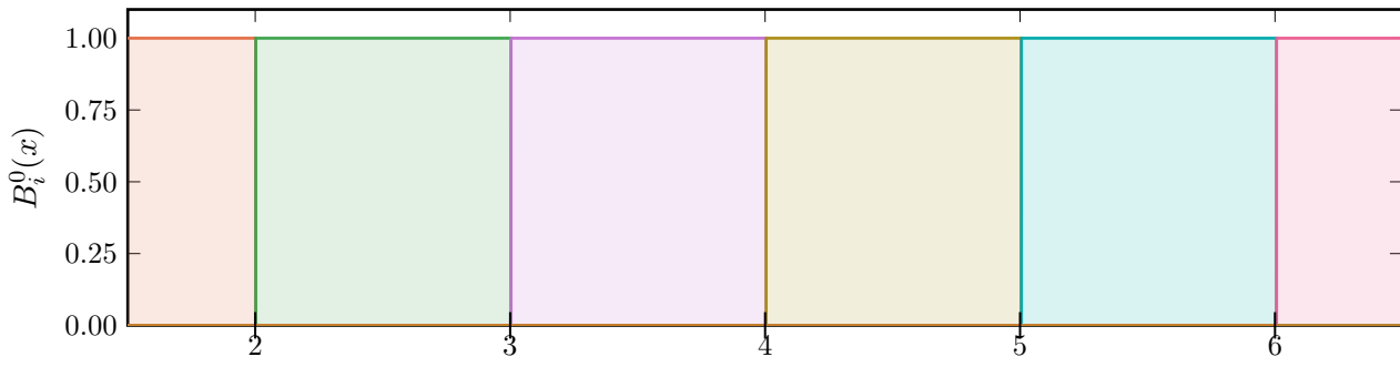
a) Grado p = 0 (Escalón)
