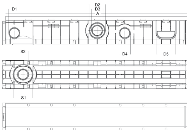
Caniveau PP bordure en plastique
