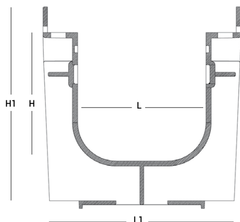
Canale PP con bordi in plastica
