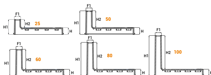
Griglia a feritoia in PP
