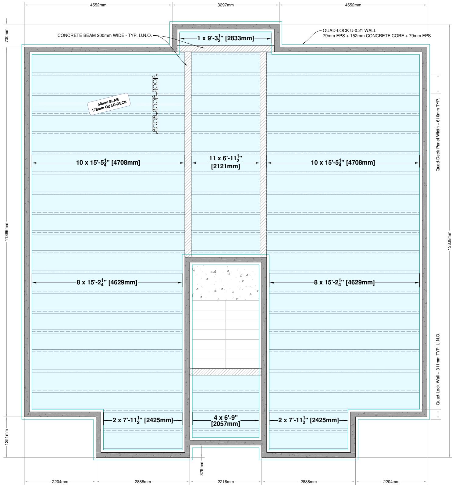
1 SECOND FLOOR PLAN Scale: N.T.S.
