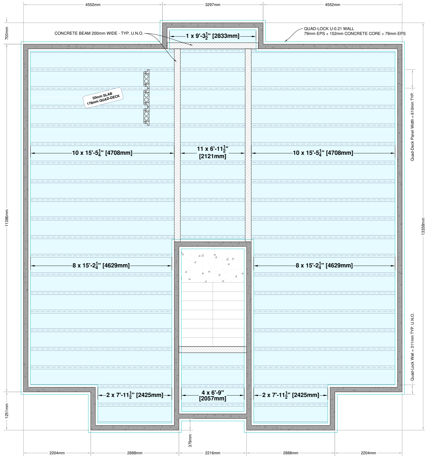
2 ROOF LEVEL PLAN Scale: N.T.S.
