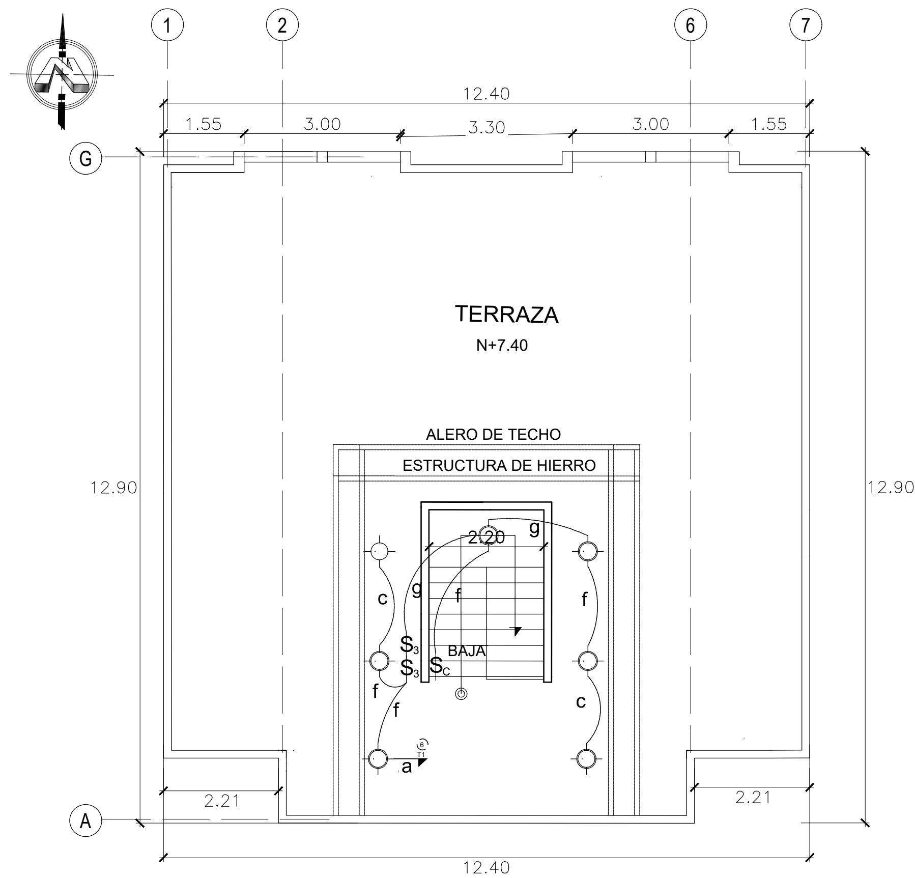
PLANTA INSTALACIONES ELECTRICAS LUCES E INTERRUPTORES TERRAZA ESC. 1:75
