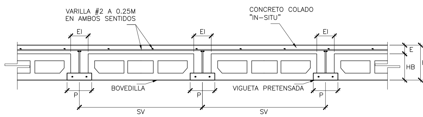
CORTE SECCION TRANSVERSAL DE LOSA ESC. 1:12.5
