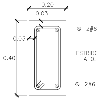
VIGA V-2 ESC. 1:10
