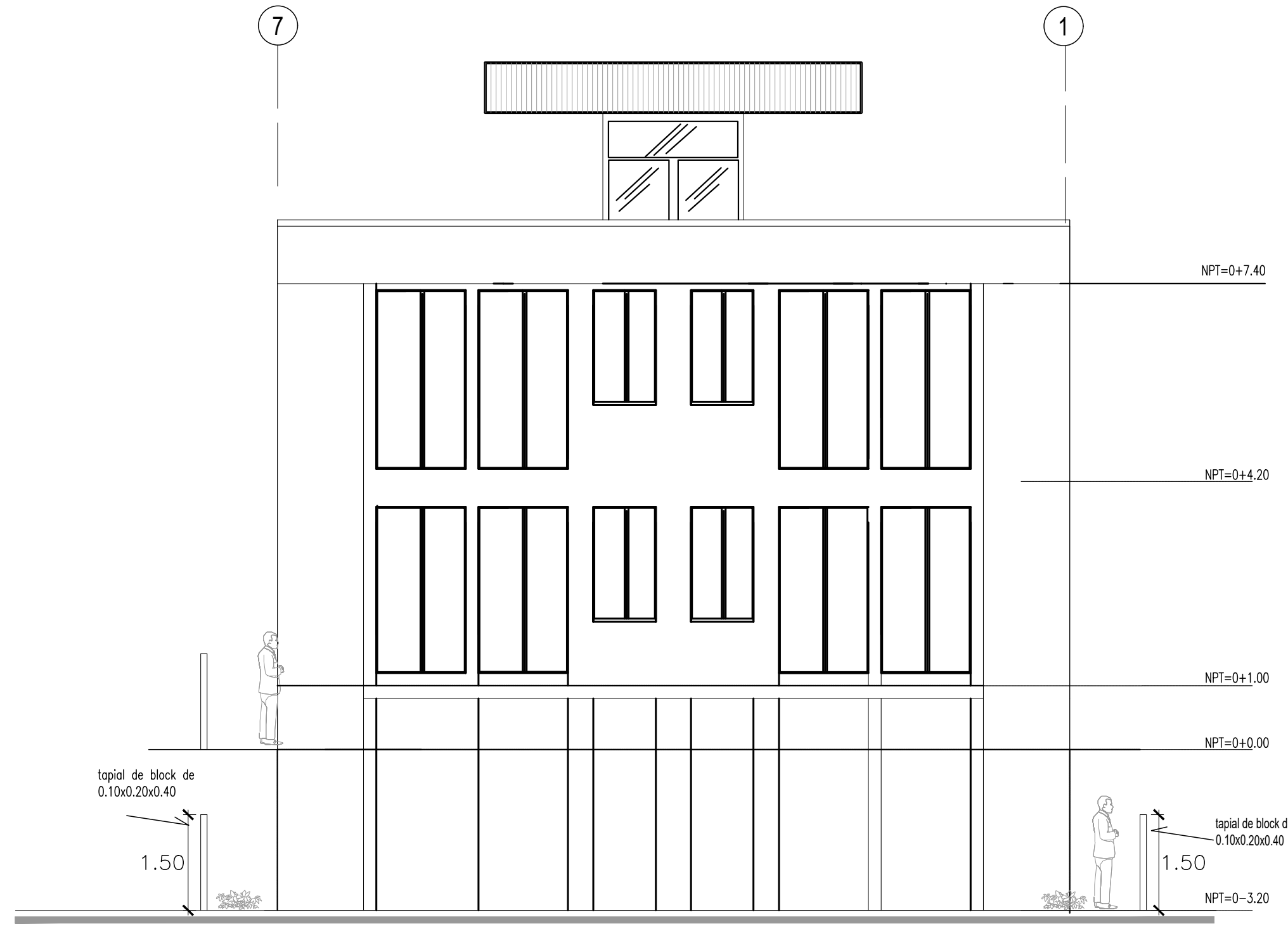
FACHADA POSTERIOR ESC. 1:75
