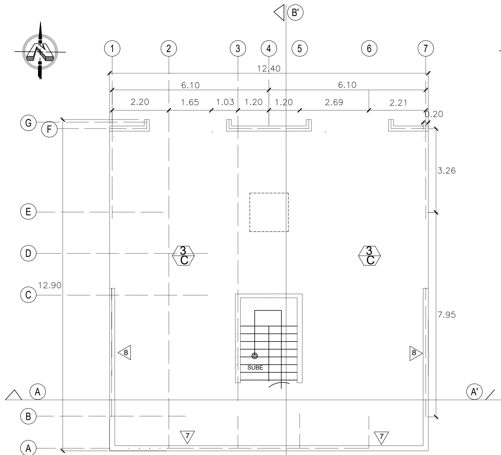
PLANTA DE ACABADOS NIVEL FUNDACION ESC. 1:75
