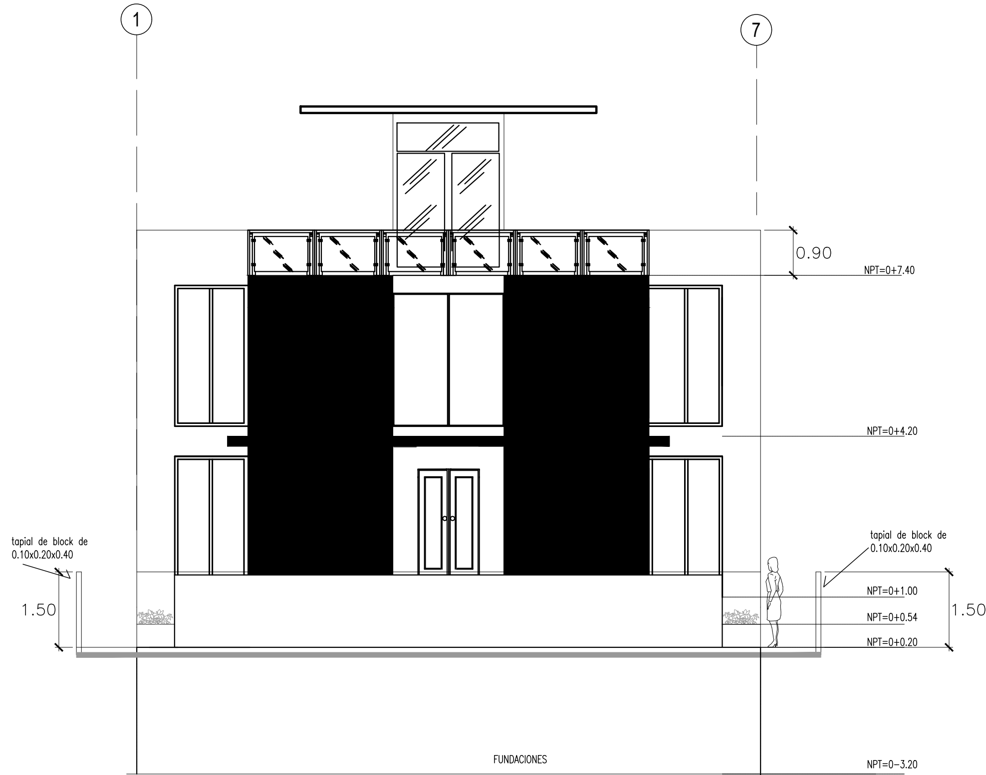
FACHADA PRINCIPAL ESC. 1:75
