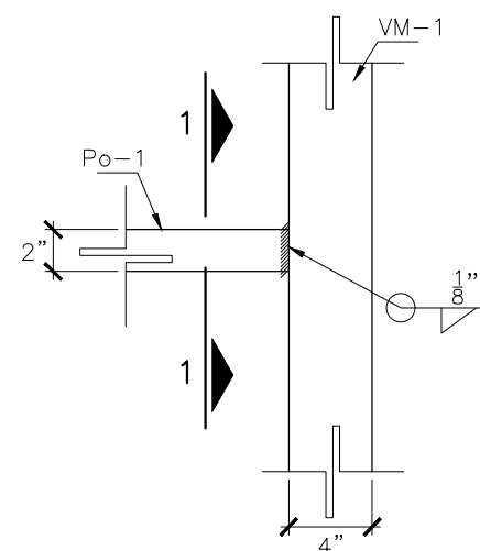
UNION VIGA A POLIN PLANTA ESC. 1:10
