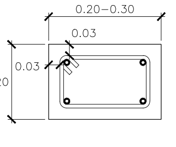
NERVIO N-2 ESC. 1:10
