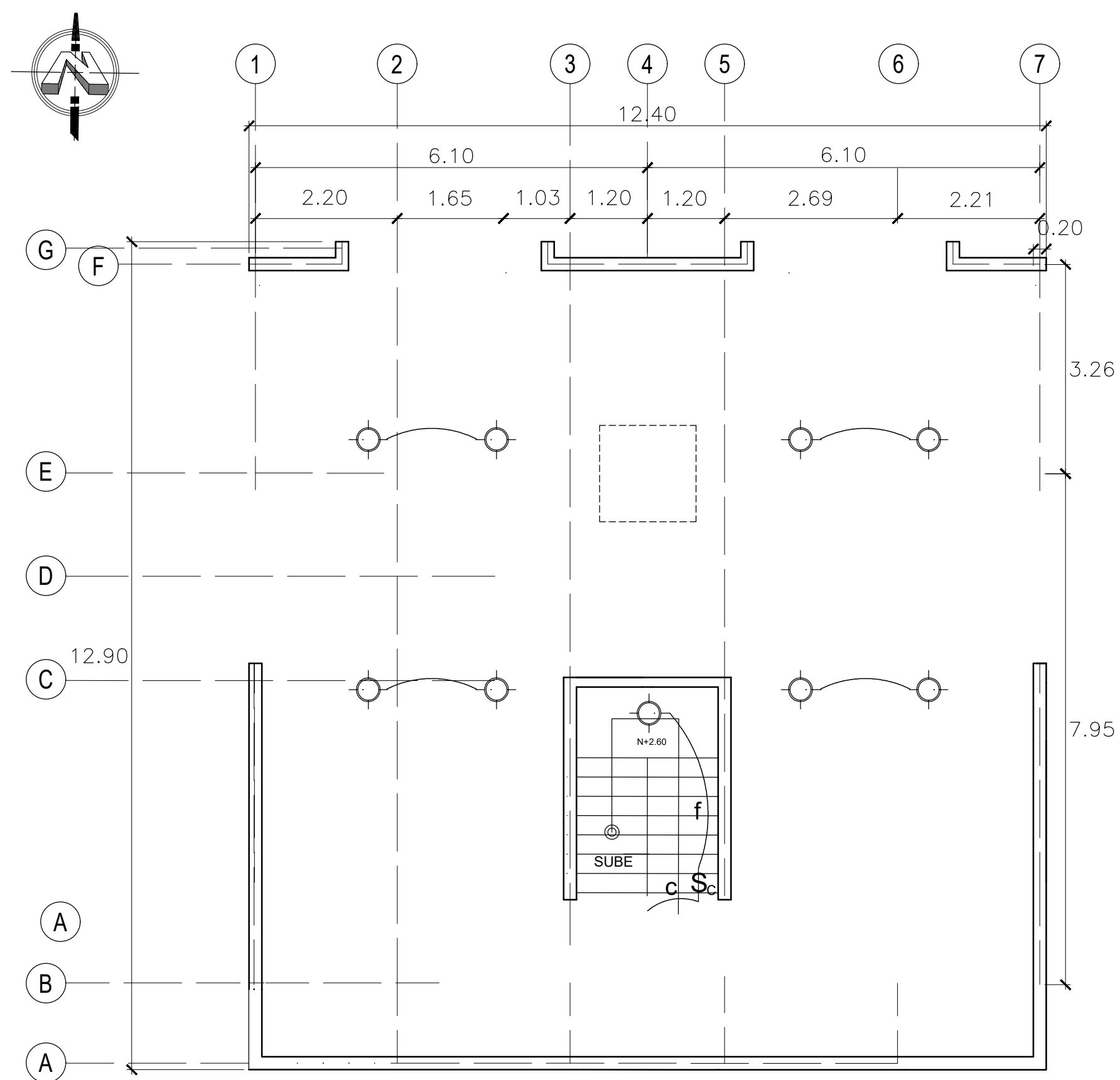
PLANTA DE INSTALACIONES ELECTRICAS LUCES E INTERRUPTORES NIVEL FUNDACION ESC. 1:75
