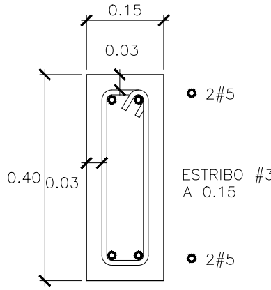
VIGA V-5 ESC. 1:10
