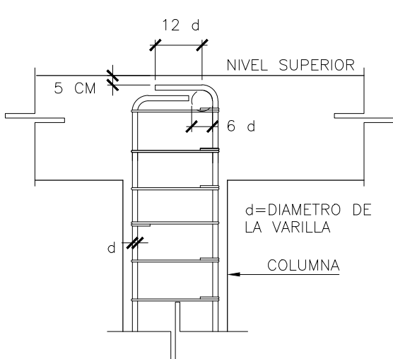
DETALLE DE REMATE EN COLUMNA ESC. 1:10
