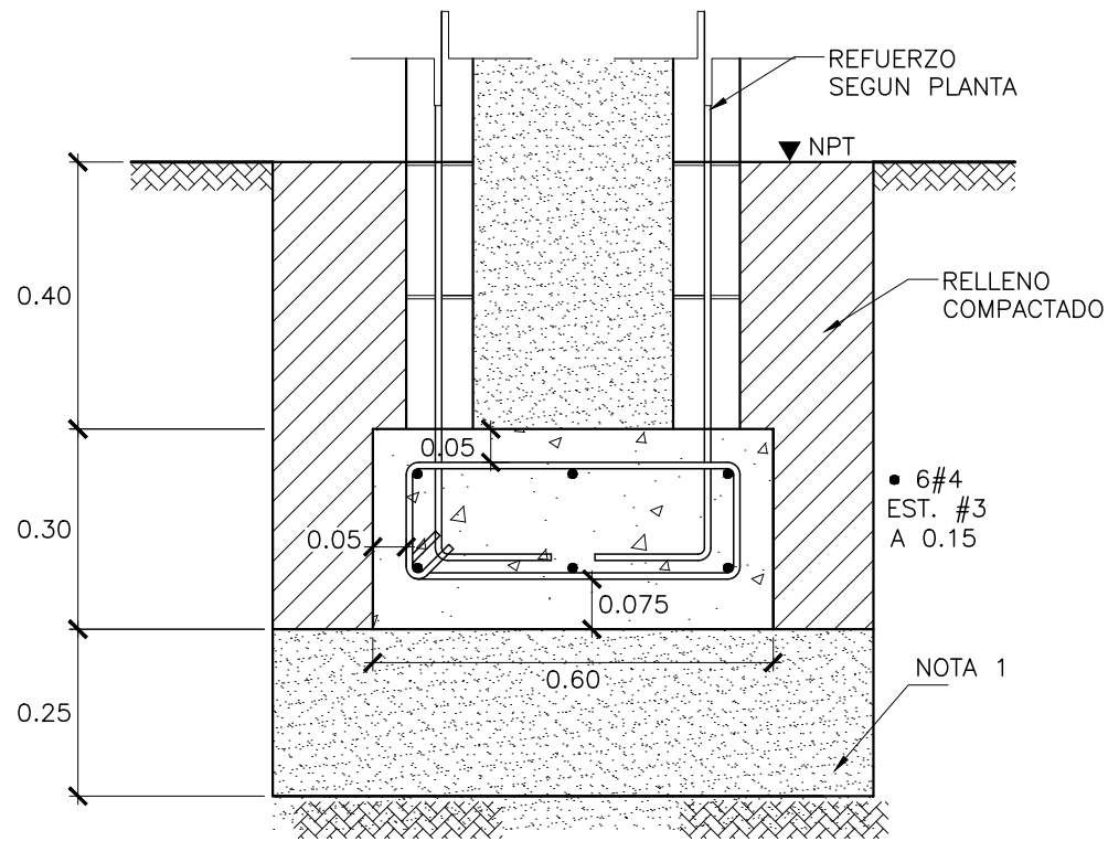
DETALLE SF-2 JARDINERA ESC. 1:12.5
