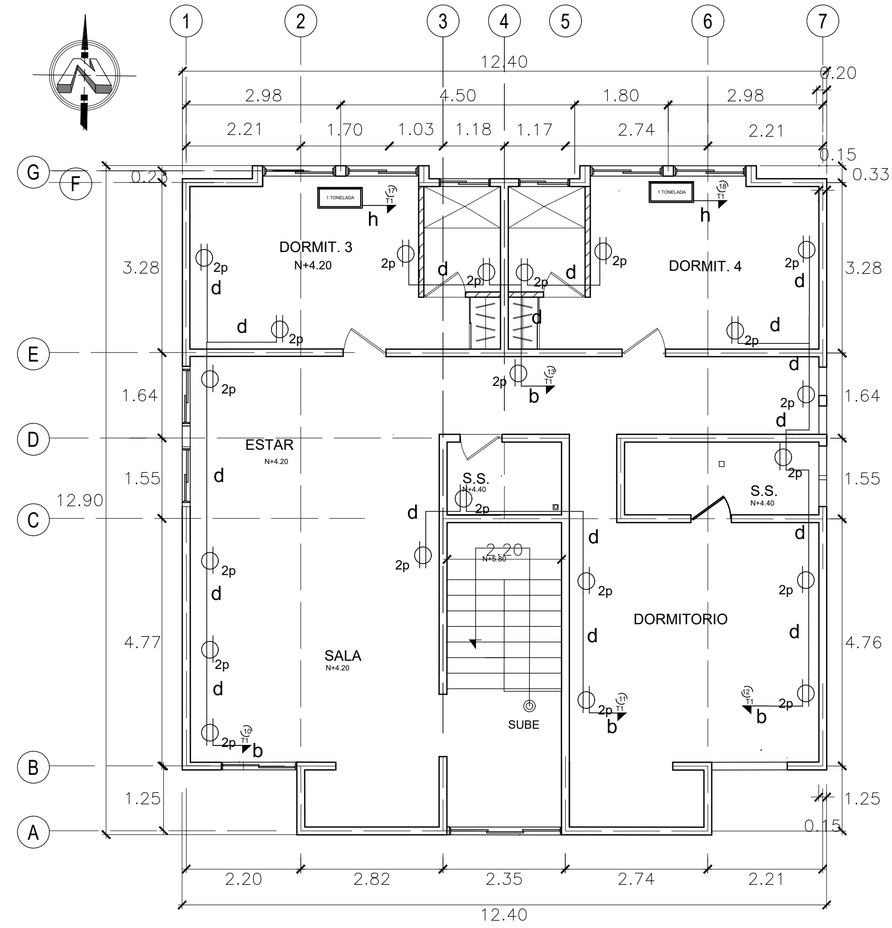
PLANTA INSTALACIONES ELECTRICAS TOMAS CORRIENTE Y A/C SEGUNDO NIVEL ESC. 1:75
