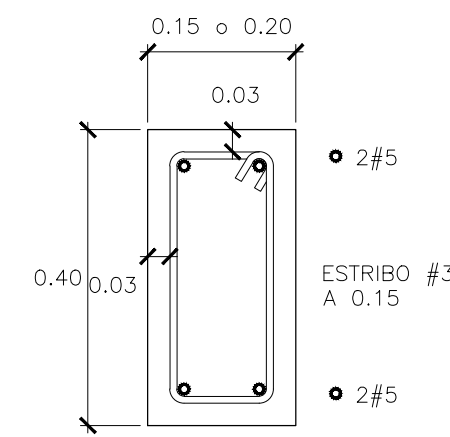
VIGA VE-1 ESC. 1:10
