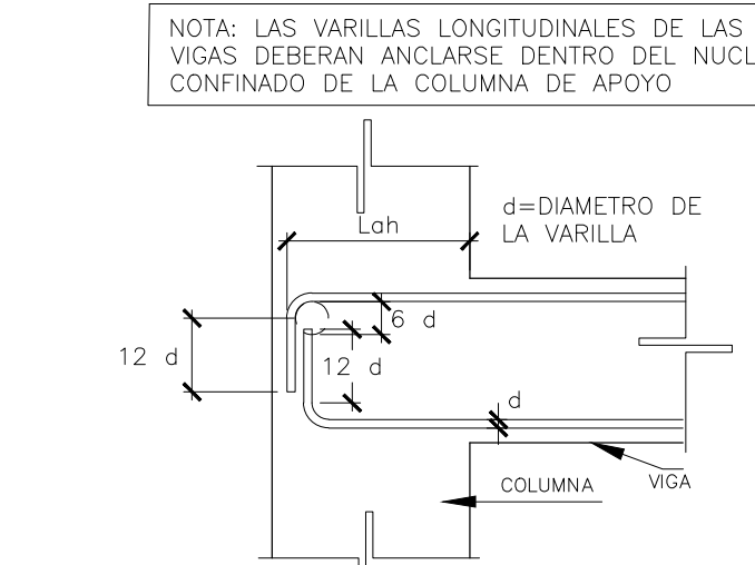
ANCLAJE DE VIGA A COLUMNAS ESC. 1:10
