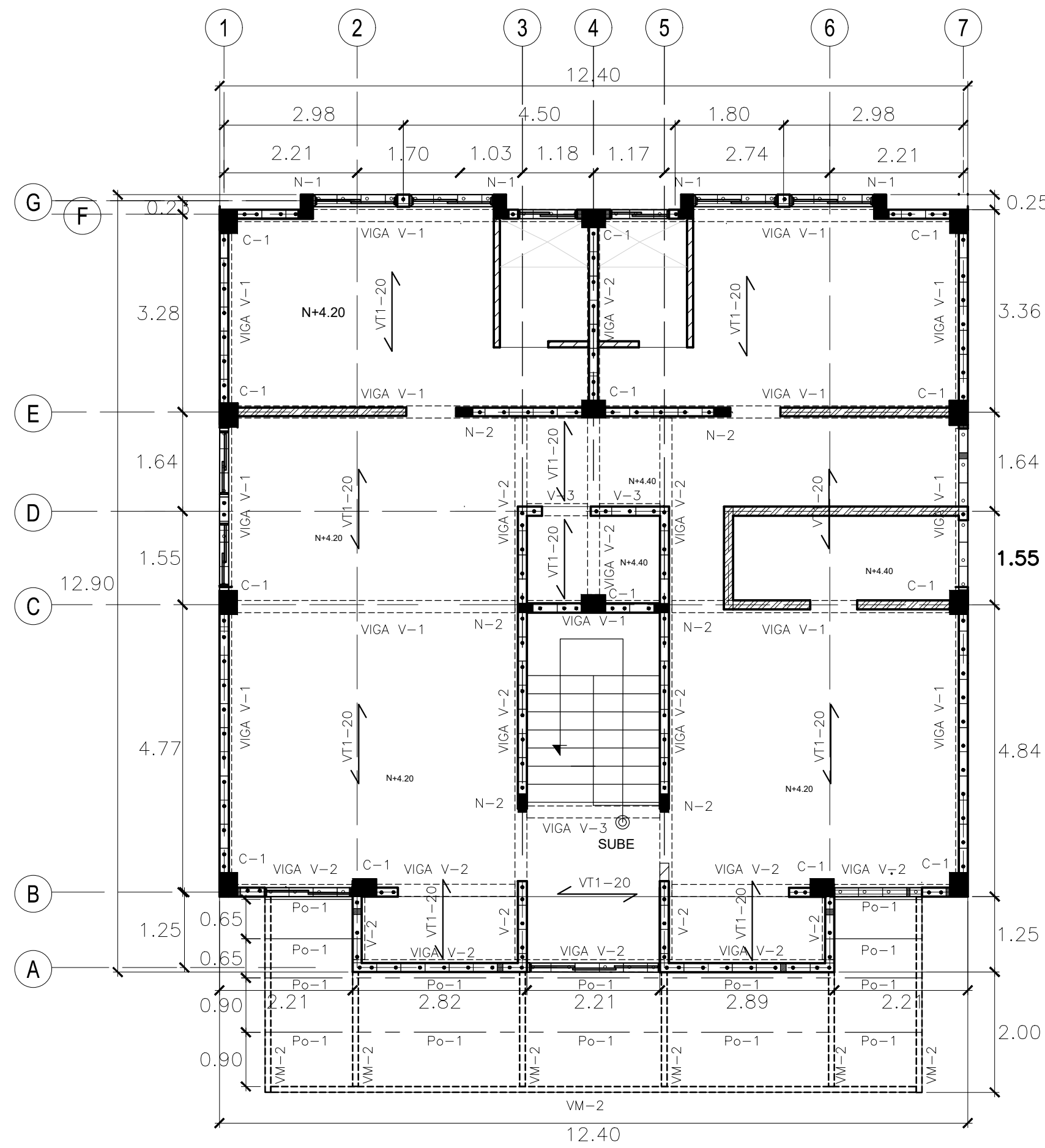
PLANTA DE ENTREPISOS SEGUNDO NIVEL ESC. 1:75
