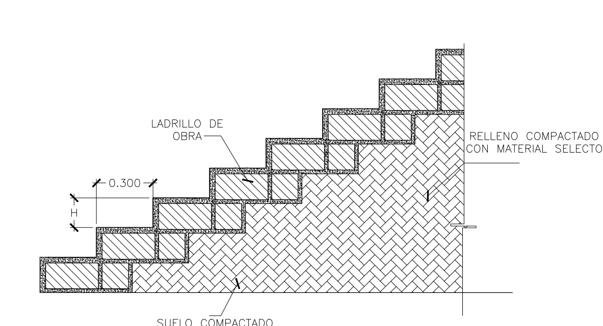
DETALLE TÍPICO DE GRADA FORJADA SIN ESCALA
