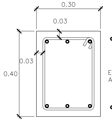
VIGA V-4 ESC. 1:10
