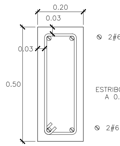
VIGA V-1 ESC. 1:10
