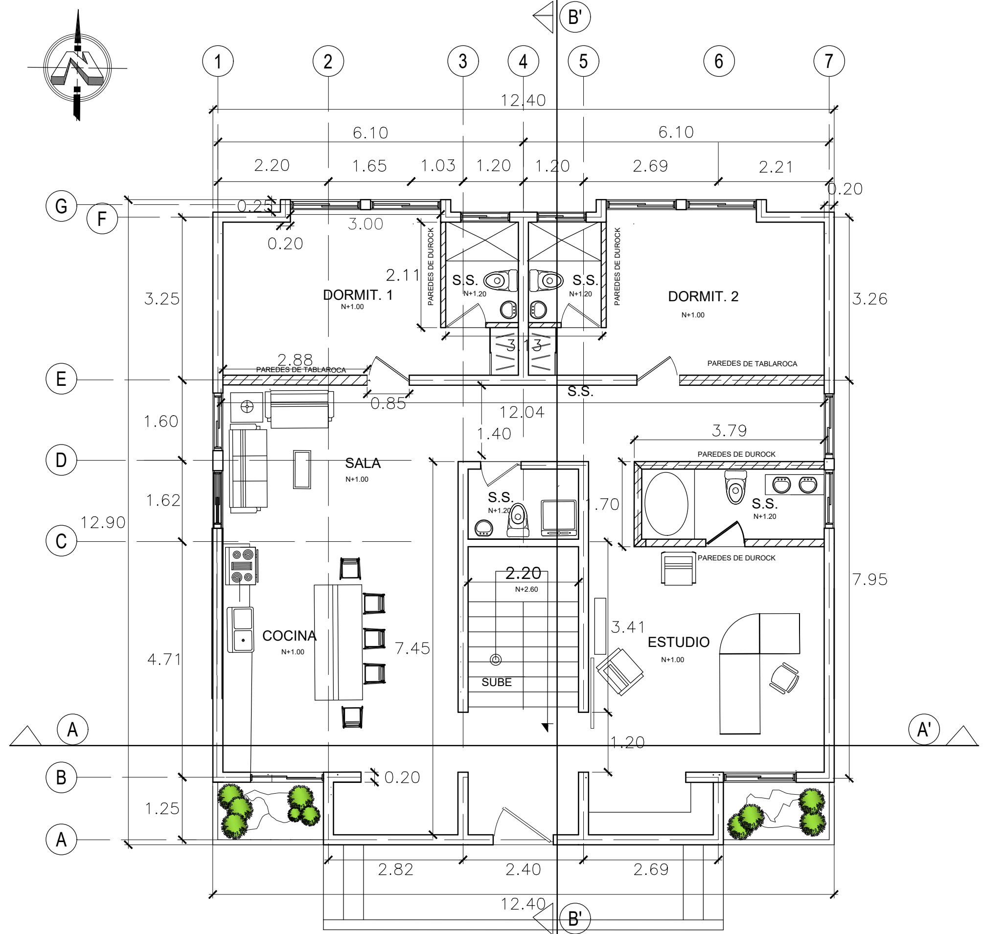
PLANTA ARQUITECTONICA PRIMER NIVEL ESC. 1:75
