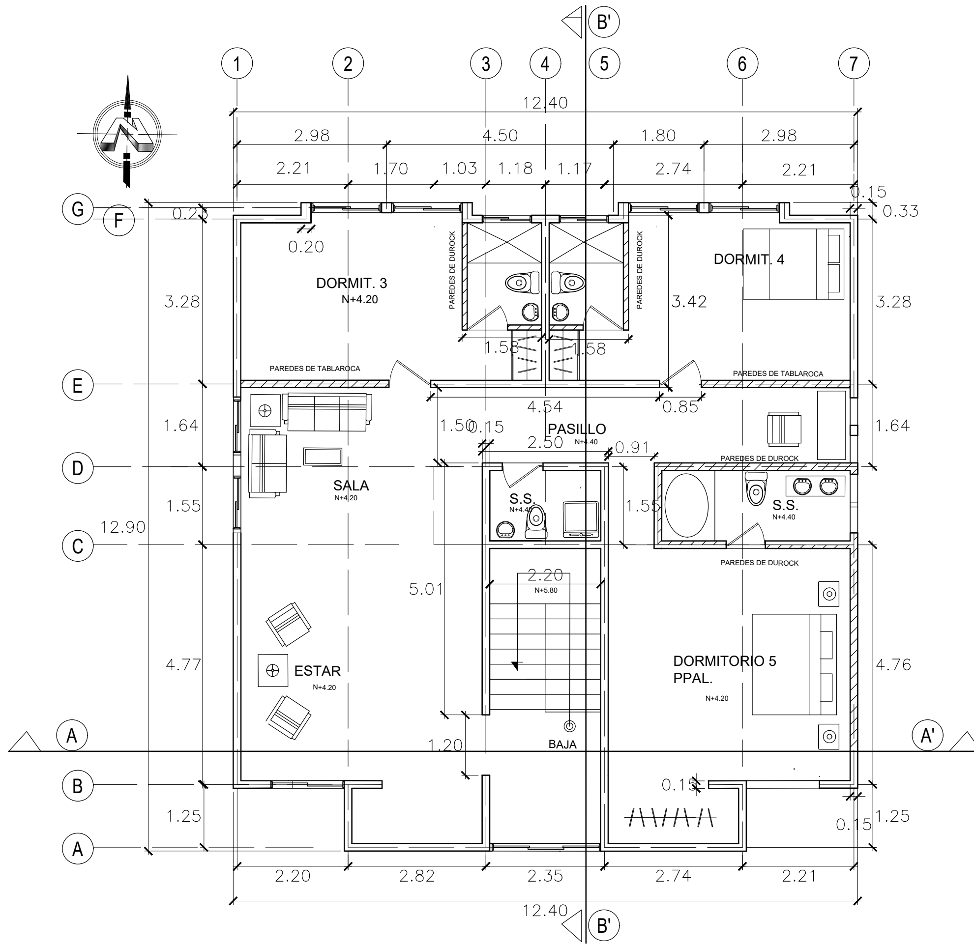
PLANTA ARQUITECTONICA SEGUNDO NIVEL ESC. 1:75
