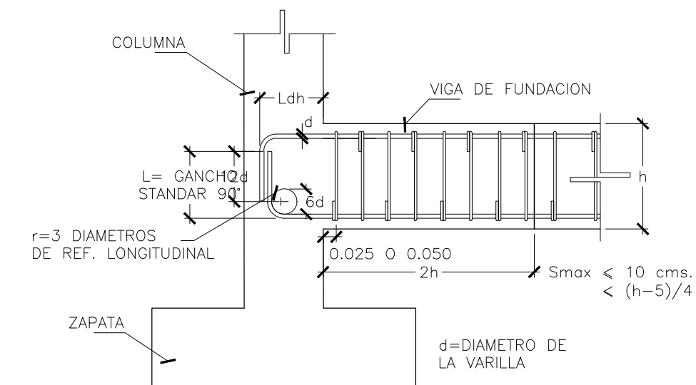
ANCLAJE FUNDACION EN COLUMNAS ESC. 1:20
