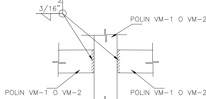
CONEXION ENTRE VIGAS METALICAS ESC. 1:10
