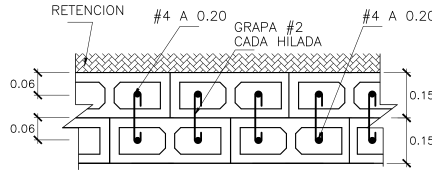
SECCION 1-1 ESC. 1:12.5
