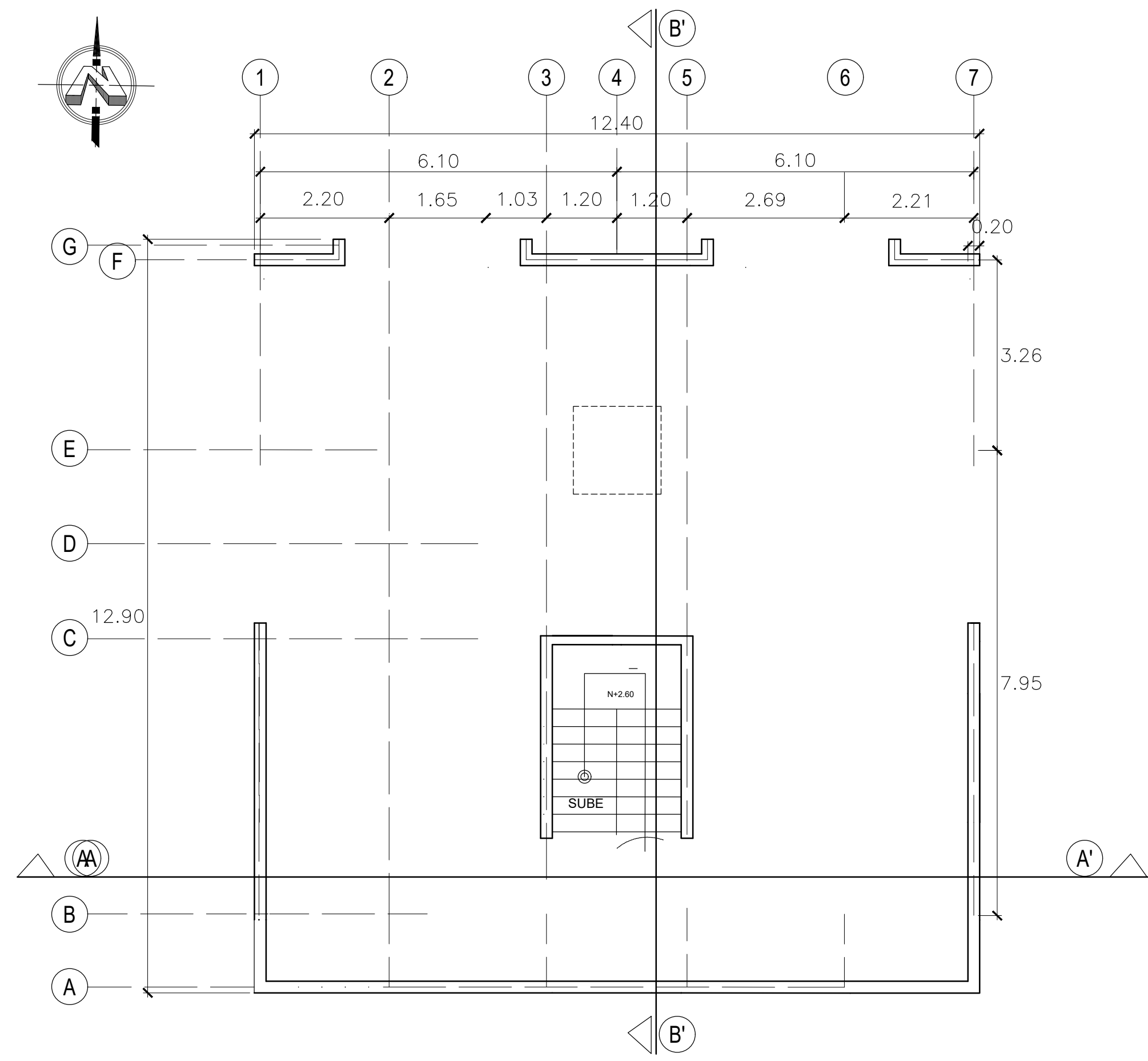
PLANTA ARQUITECTONICA NIVEL FUNDACION ESC. 1:75
