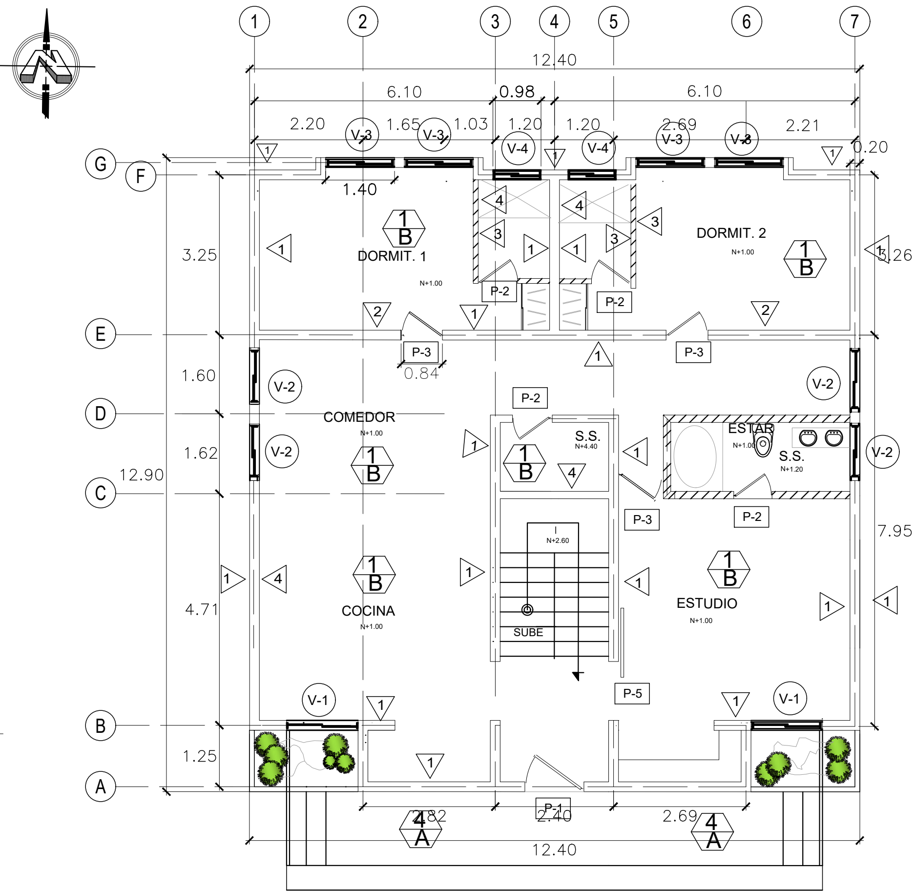
PLANTA DE ACABADOS PRIMER NIVEL ESC. 1:75
