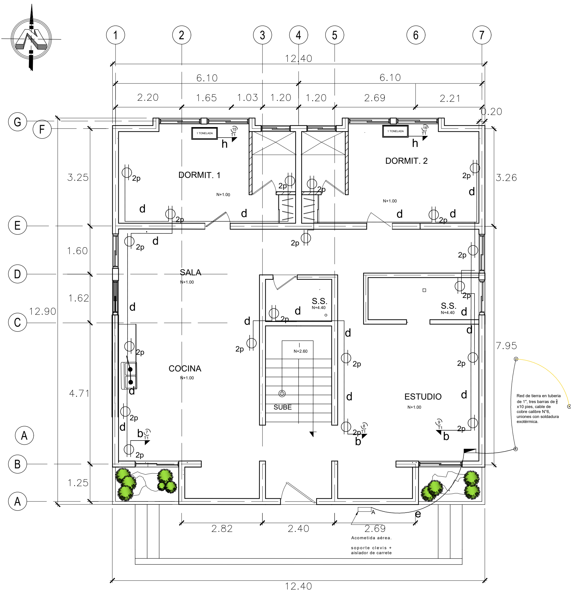
PLANTA DE INSTALACIONES ELECTRICAS TOMAS CORRIENTE Y A/C PRIMER NIVEL ESC. 1:75
