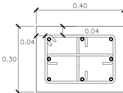
COLUMNA C-1 ESC. 1:10
