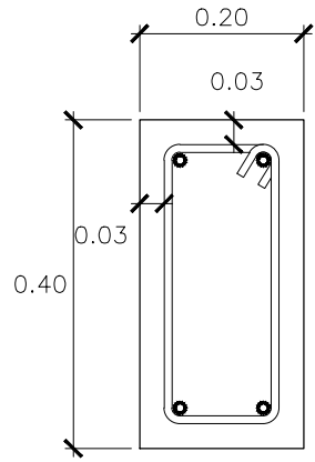
VIGA V-3 ESC. 1:10
