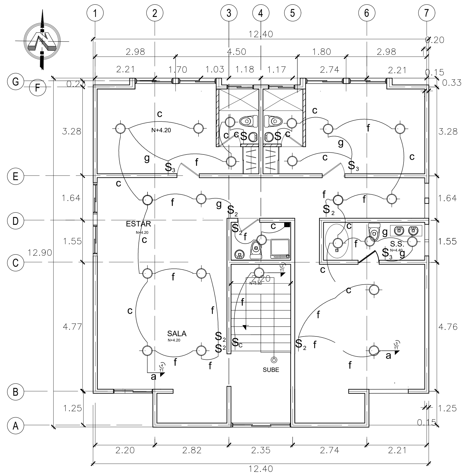
PLANTA DE INSTALACIONES ELECTRICAS LUCES E INTERRUPTORES SEGUNDO NIVEL ESC. 1:75
