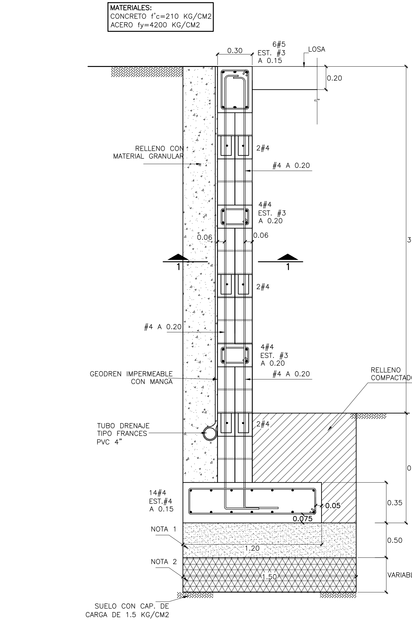
MURO MB-1 ESC. 1:12.5
