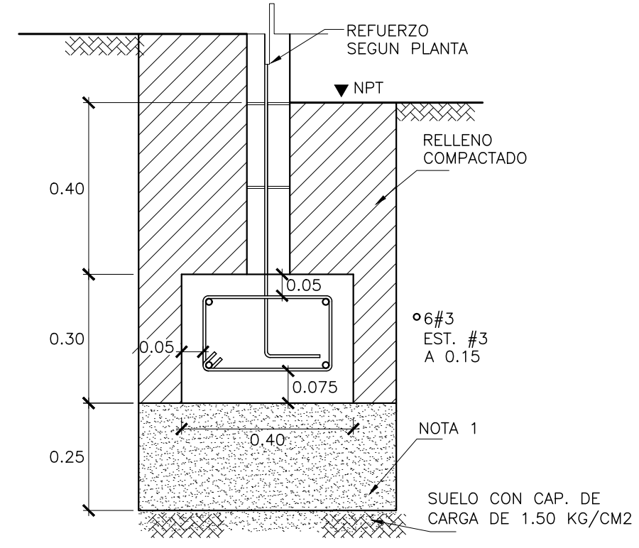
DETALLE SF-3 JARDINERA ESC. 1:12.5
