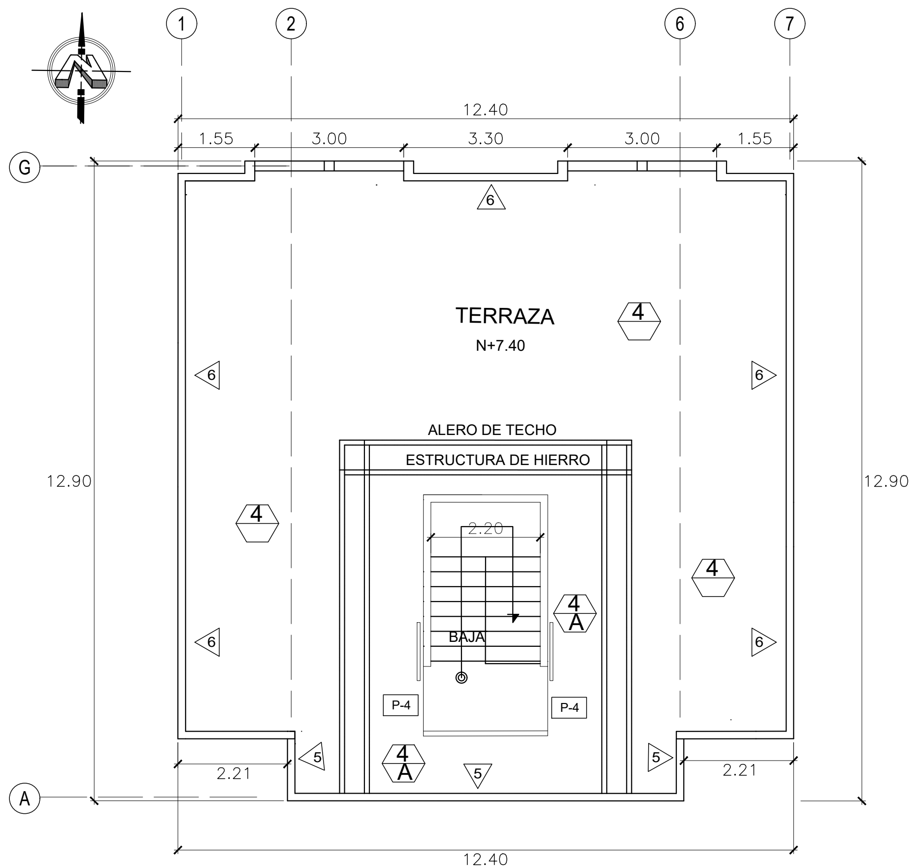
PLANTA ACABADOS TERRAZA ESC. 1:75
