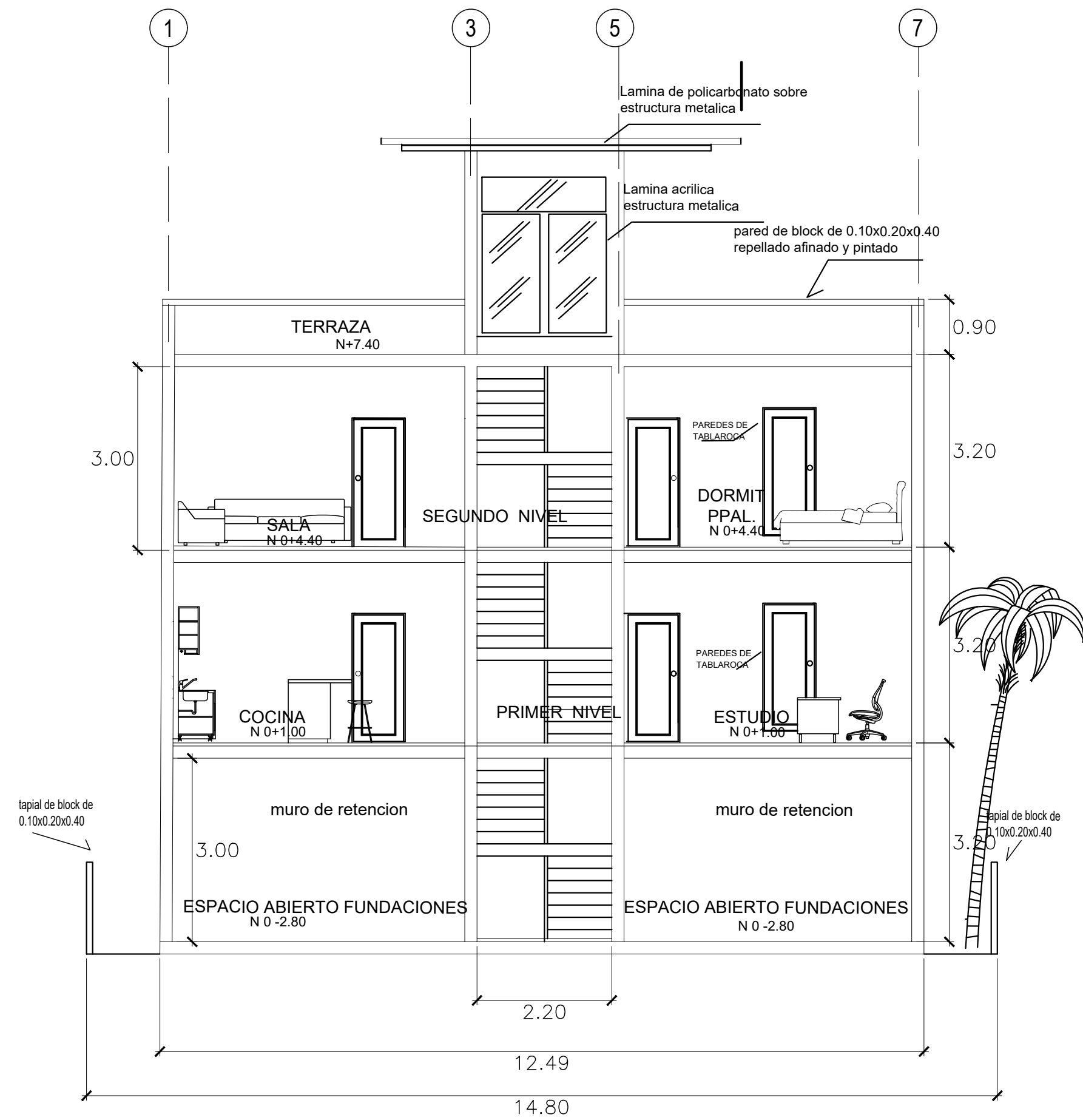
SECCION A A' ESC. 1:75
