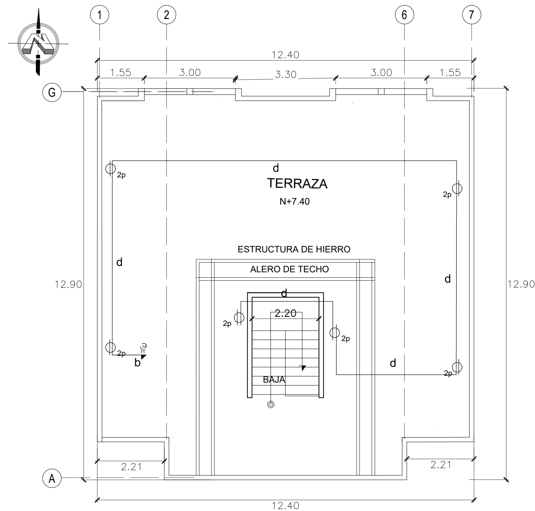
PLANTA INSTALACIONES ELECTRICAS TOMAS CORRIENTE TERRAZA
