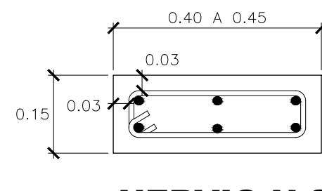
NERVIO N-3 ESC. 1:10
