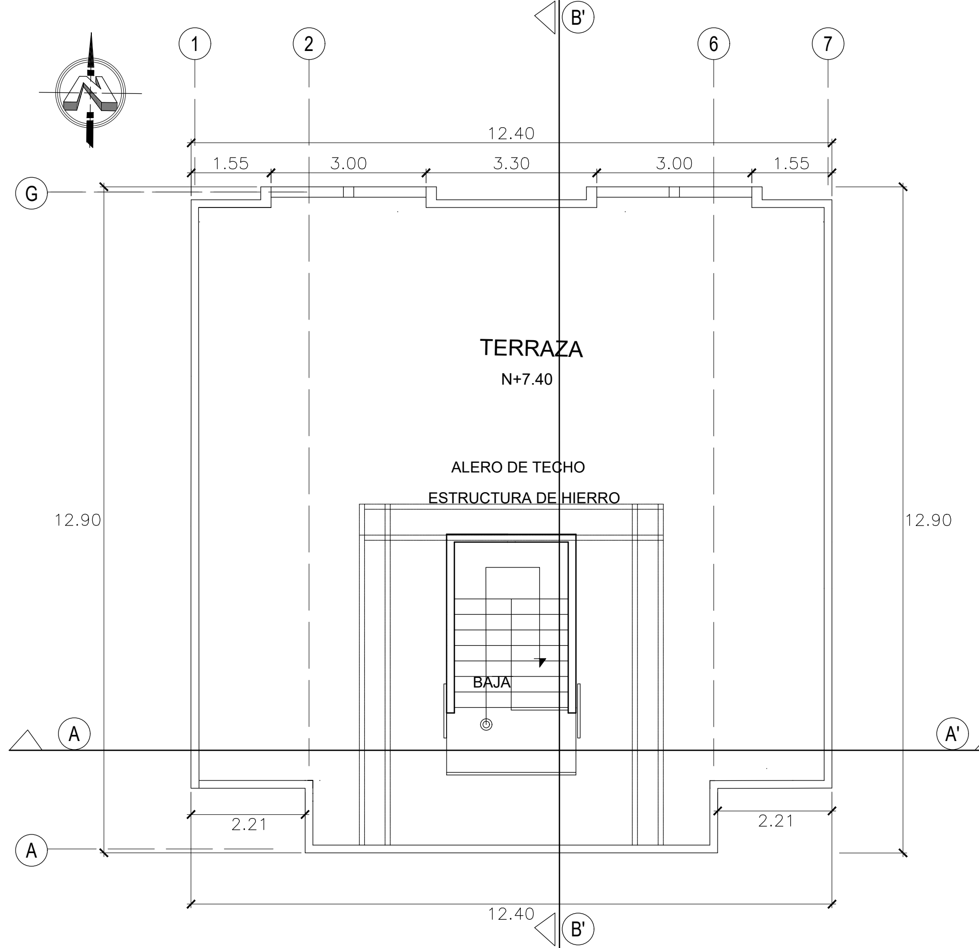
PLANTA ARQUITECTONICA TERRAZA ESC. 1:75
