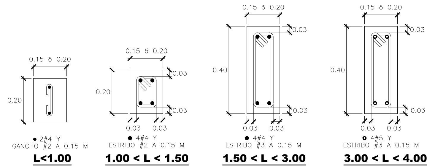
DETALLES DE CARGADEROS ESC. 1:10
