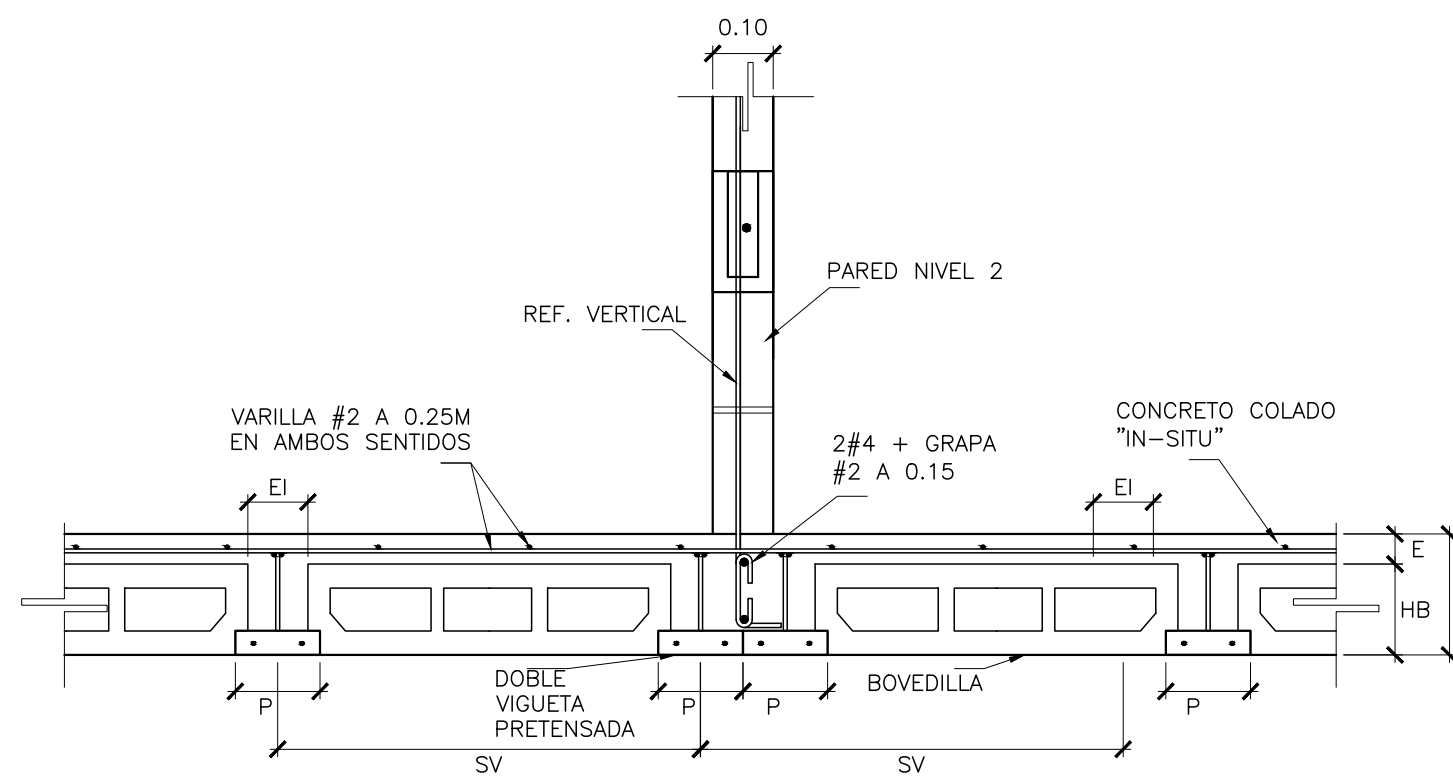
APOYO DE PARED SOBRE LOSA - PARED PARALELA A VIGUETA ESC. 1:12.5
