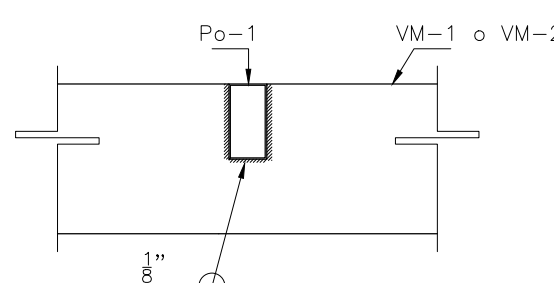
SECCION 1-1 ELEVACION ESC. 1:10
