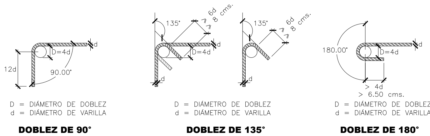
DETALLES DE DOBLECES DE REFUERZO EN ESTRIBOS (VARILLAS MENORES AL #5) SIN ESCALA
