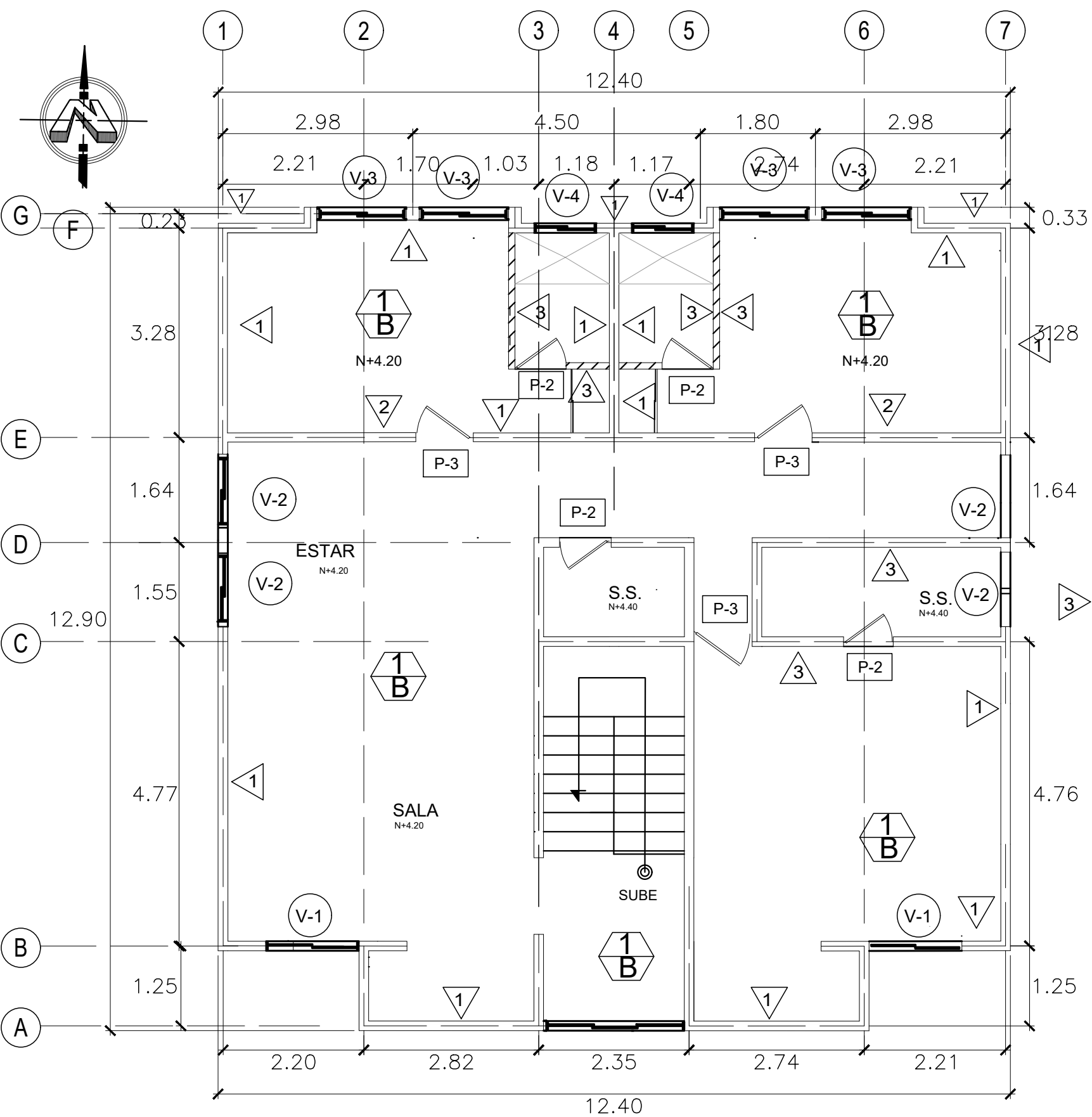
PLANTA ACABADOS SEGUNDO NIVEL ESC. 1:75
