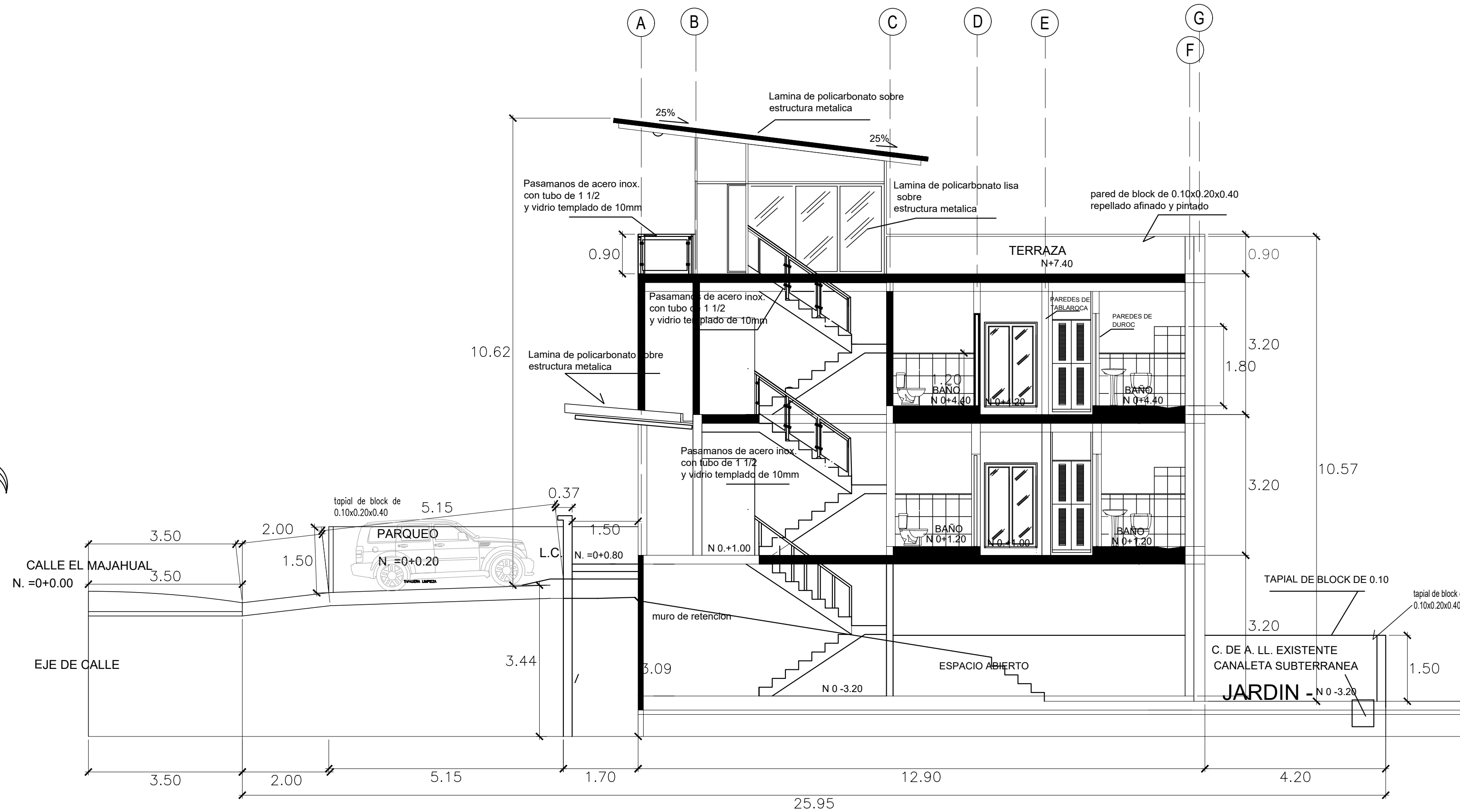
SECCION B B' ESC. 1:75
