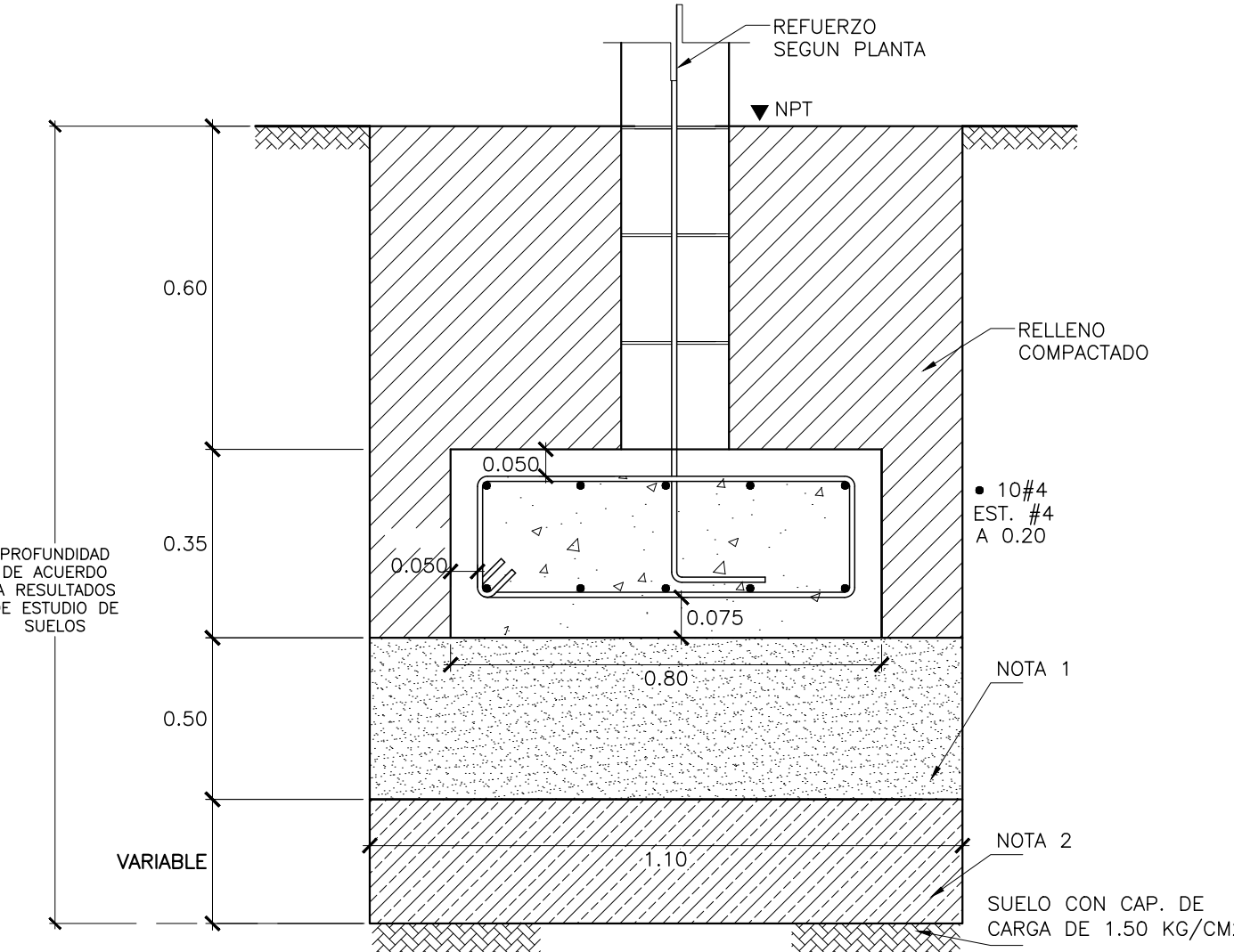
DETALLE SF-1 ESC. 1:12.5
