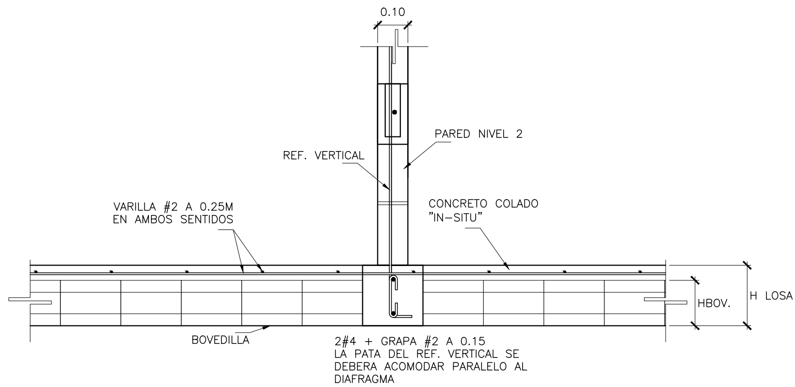
APOYO DE PARED SOBRE LOSA - PARED PERPENDICULAR A VIGUETA ESC. 1:12.5
