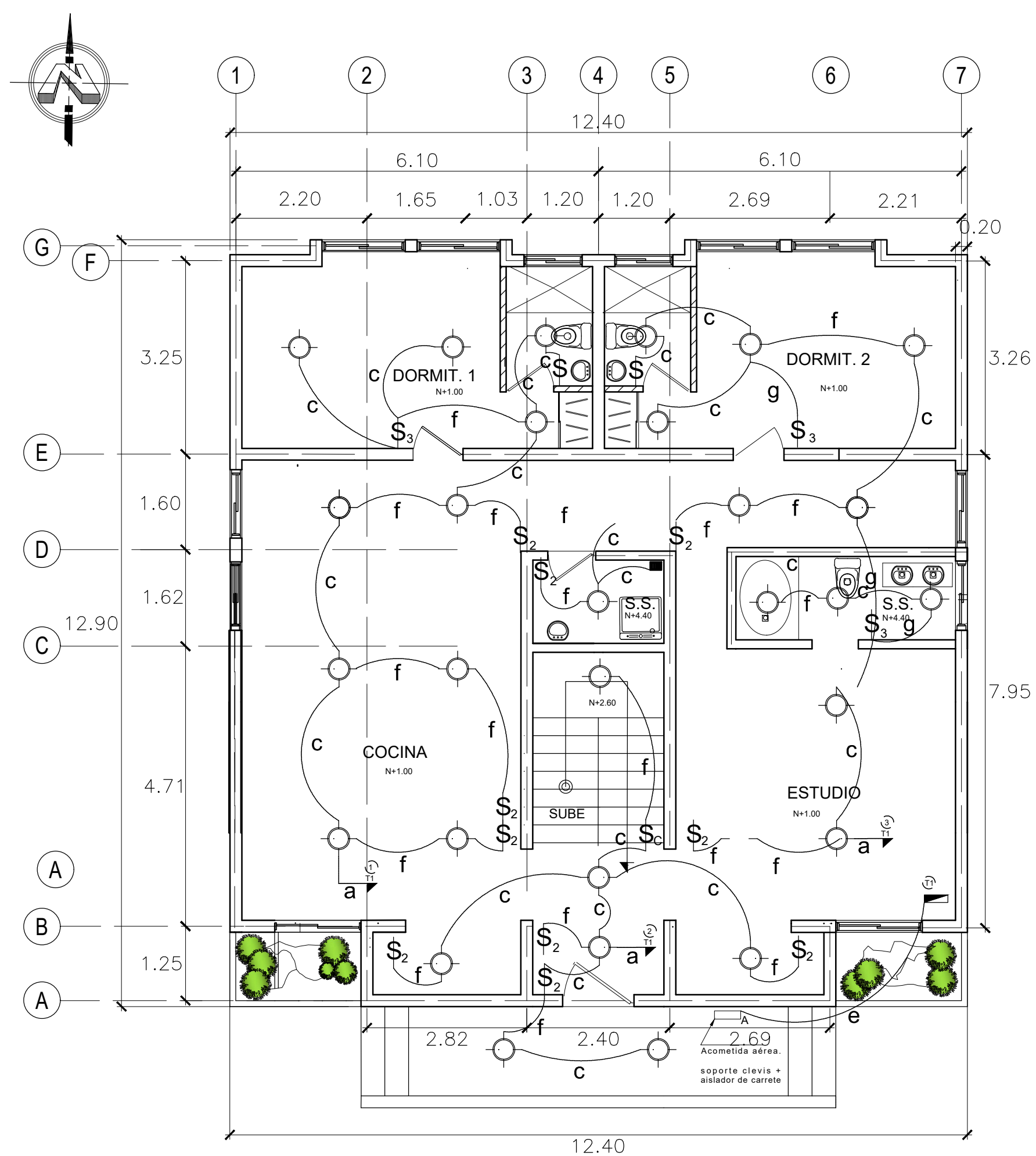
PLANTA DE INSTALACIONES ELECTRICAS LUCES E INTERRUPTORES PRIMER NIVEL ESC. 1:75
