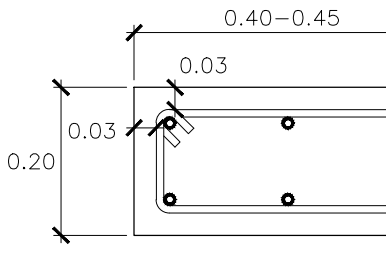
NERVIO N-1 ESC. 1:10
