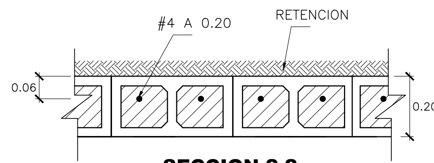
SECCION 2-2 ESC. 1:12.5
