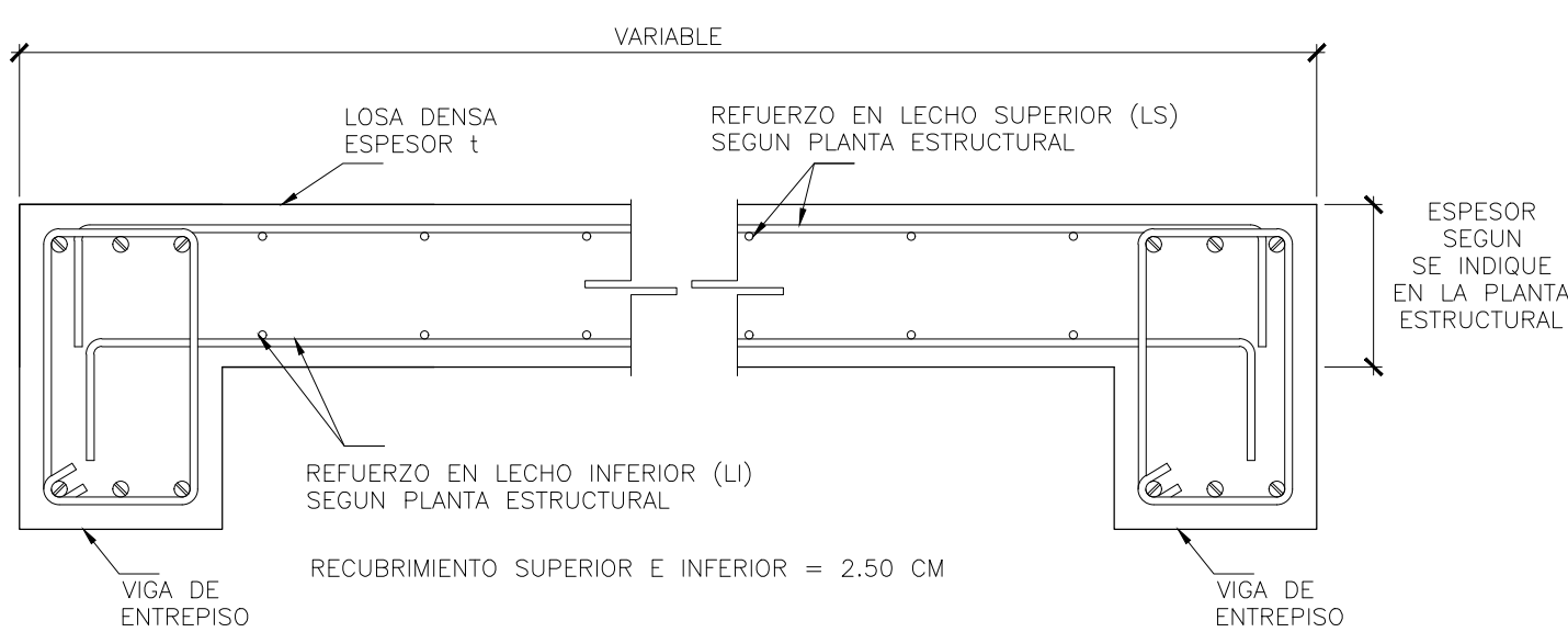
SECCION TÍPICA DE LOSA Densa ESC. 1:10
