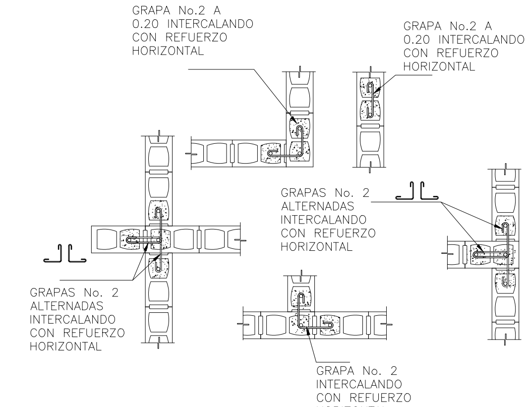
DETALLE DE UNIONES ENTRE PAREDES DE BLOQUE SIN ESCALA
