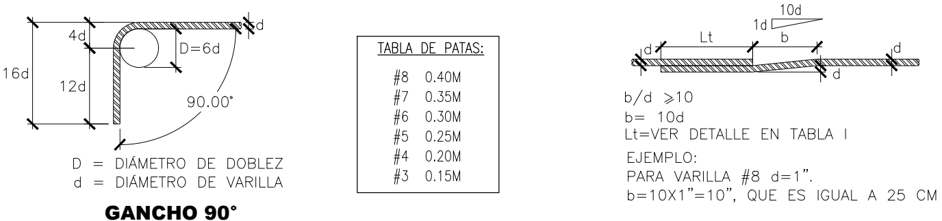
DETALLES DE DOBLEZ DE REFUERZO PRINCIPAL SIN ESCALA
