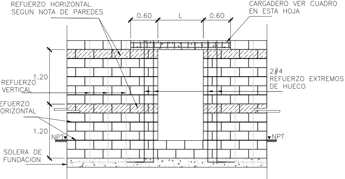
DETALLE TÍPICO DE SOLERAS INTERMEDIAS, CARGADEROS Y REPISAS SIN ESCALA
