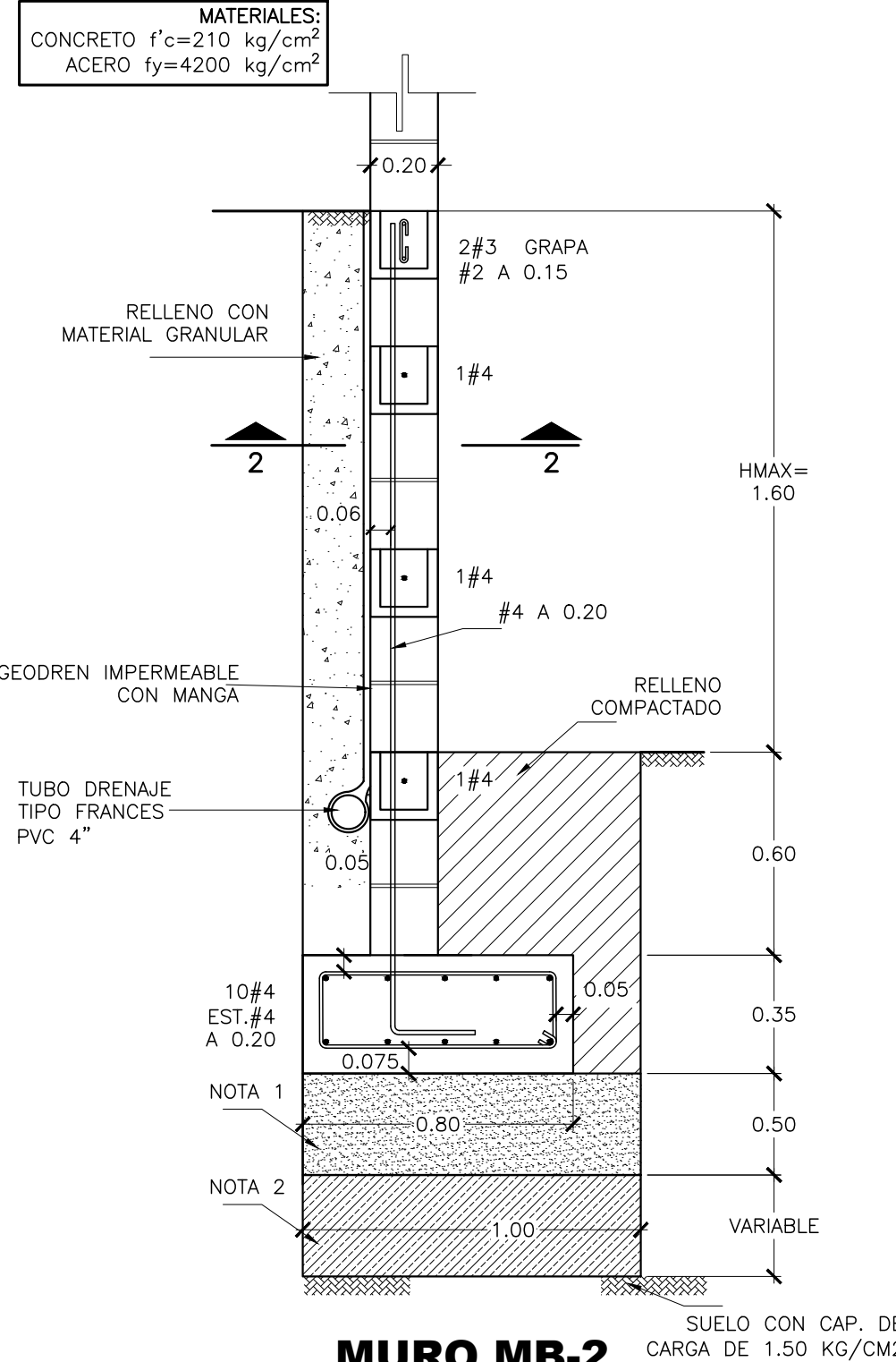
MURO MB-2 ESC. 1:20
