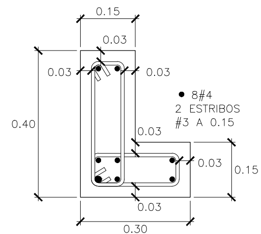
NERVIO N-4 ESC. 1:10
