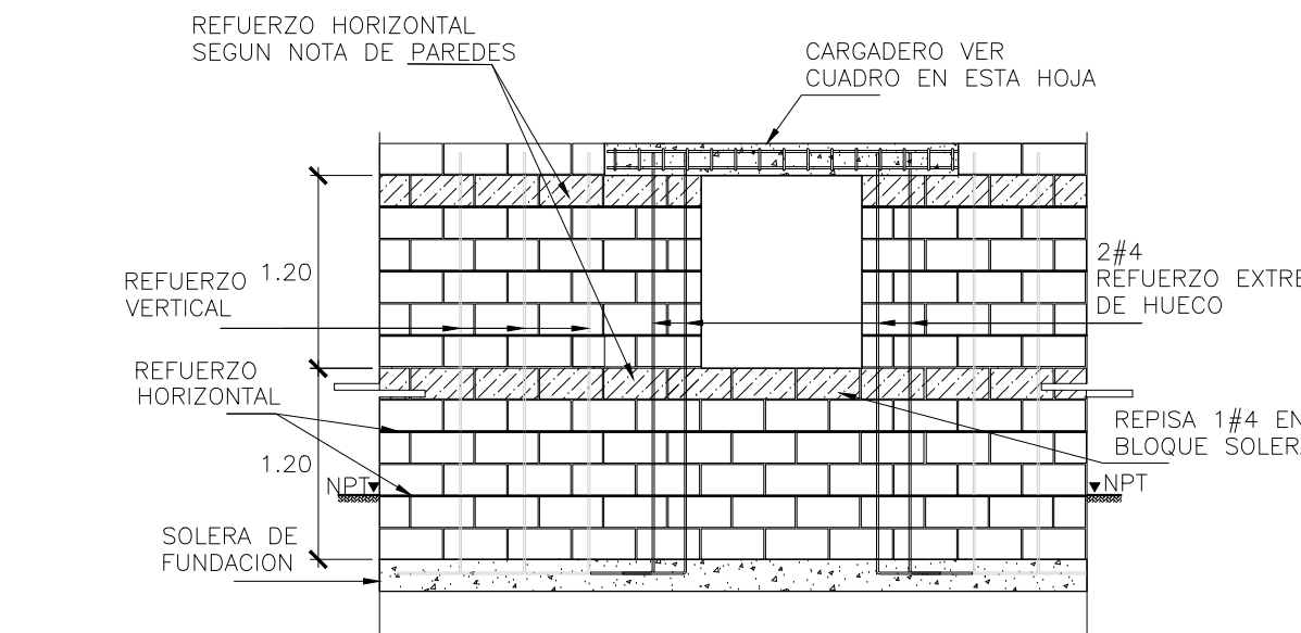
DETALLE TÍPICO DE SOLERAS INTERMEDIAS, CARGADEROS Y REPISAS SIN ESCALA
