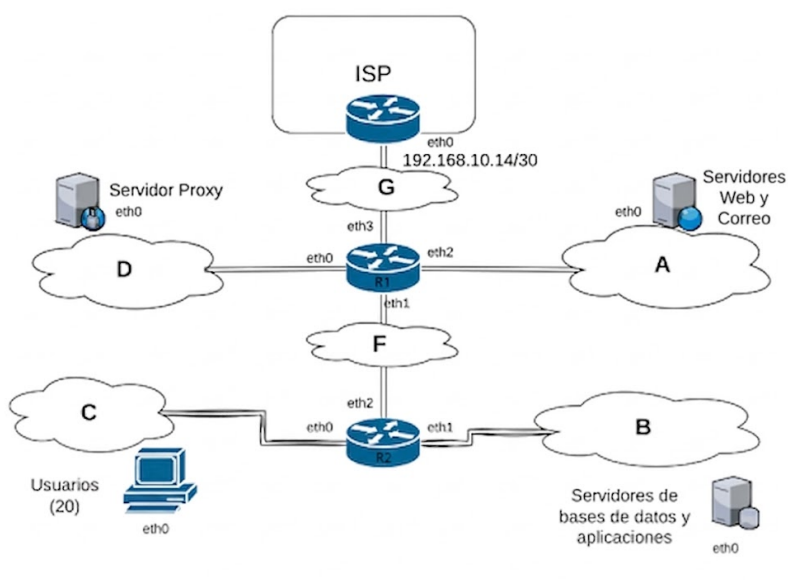
Figura 1: Topología de la red de la organización
