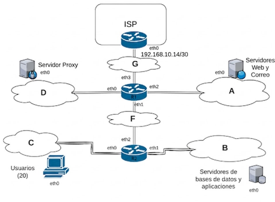
Figura 1: Topología de la red de la organización
