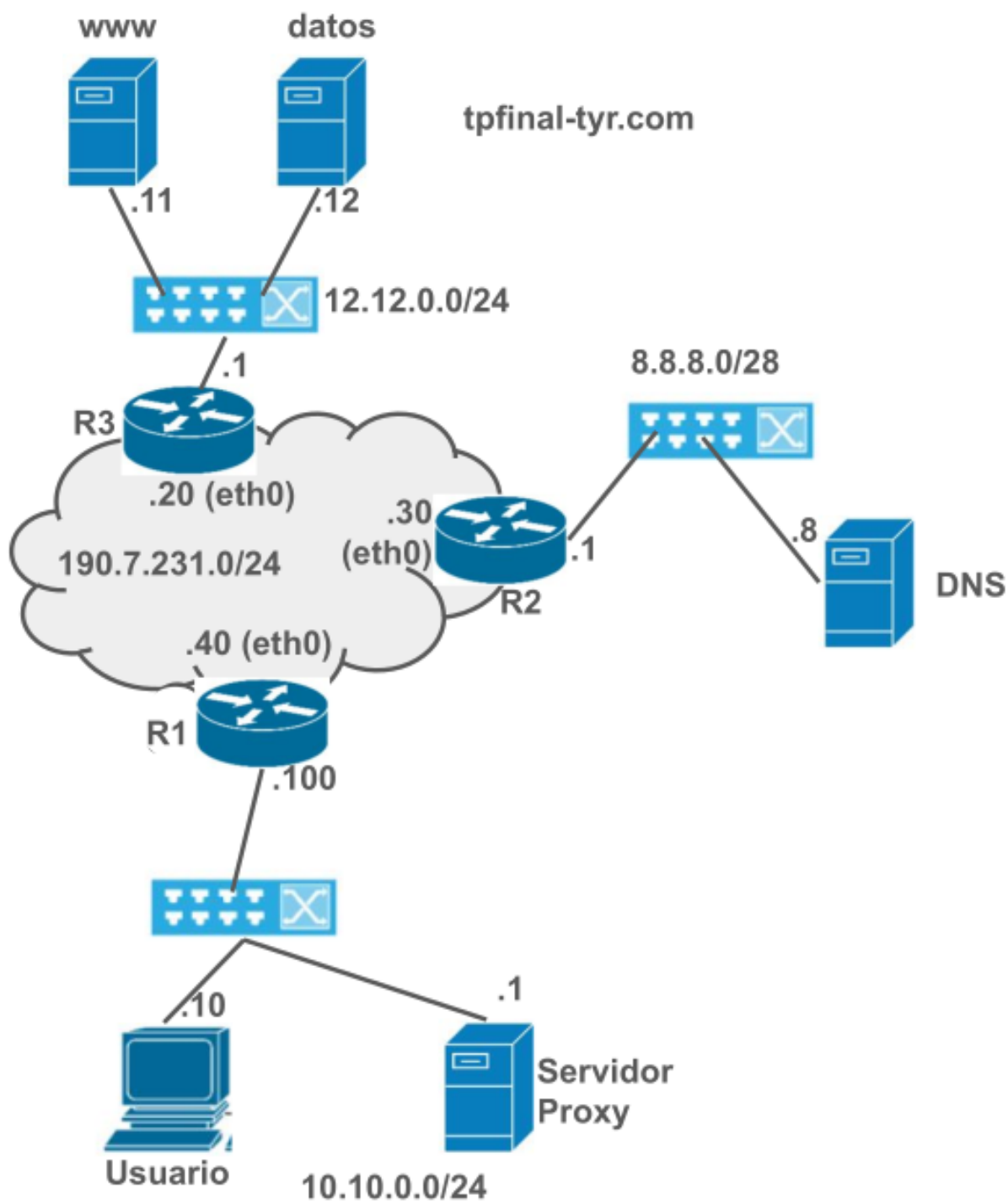
Figura 1: Topología
