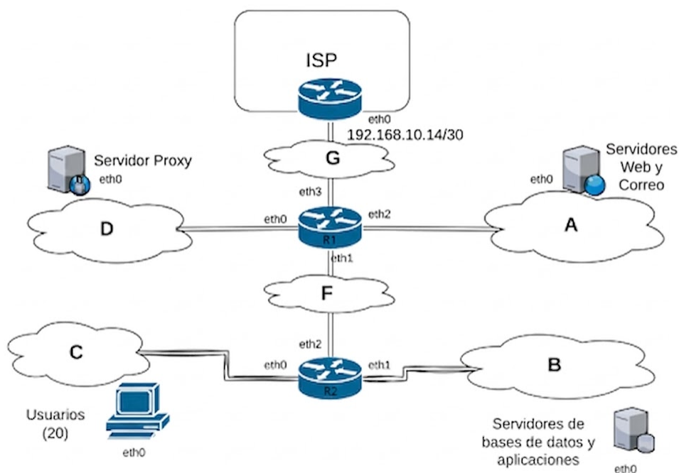
Figura 1: Topología de la red de la organización
