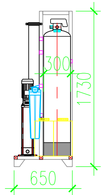
右视图 (Right View)
