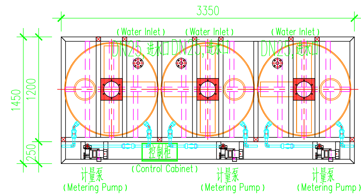
俯视图 (Top View)
