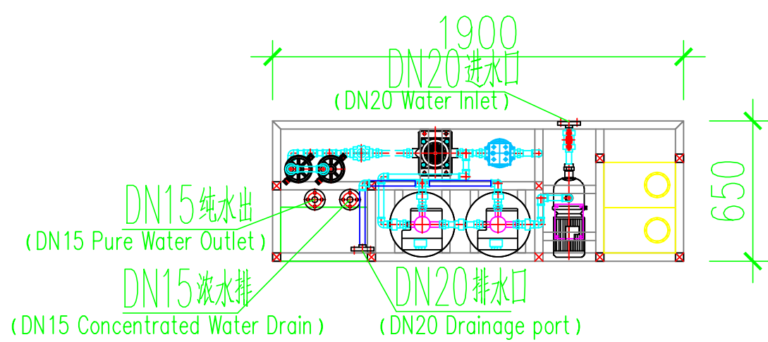
俯视图 (Top View)
