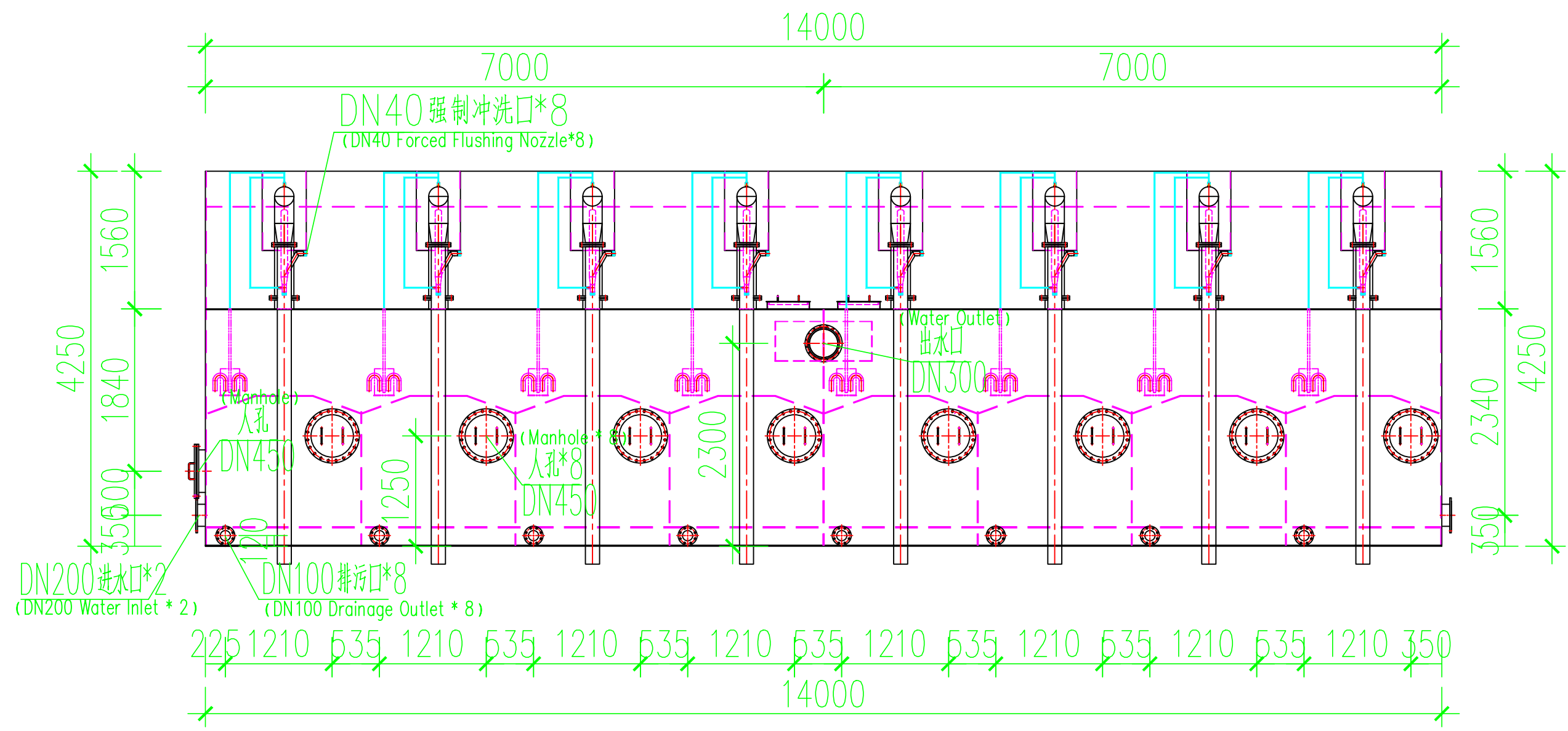
正视图 (Front View)
