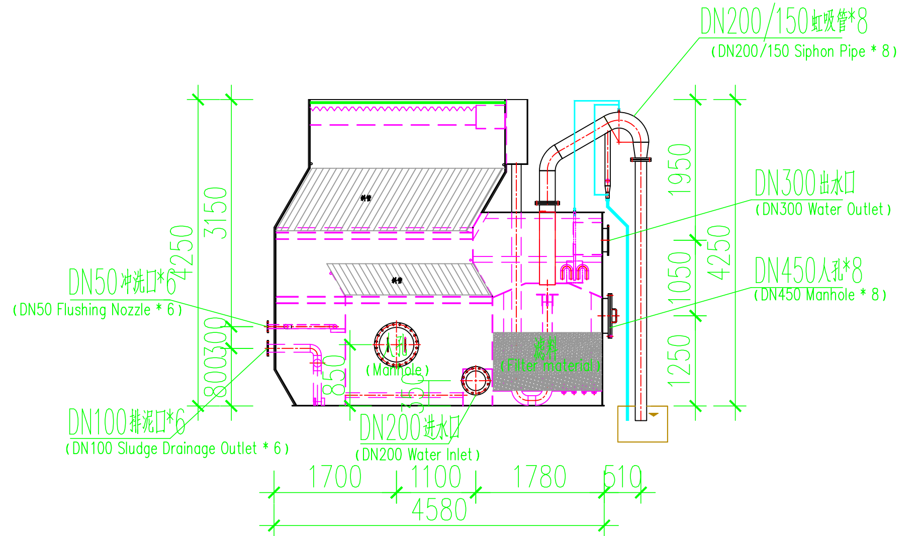
左视图 (Left View)
