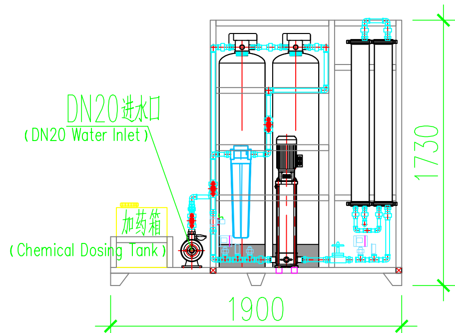
后视图 (Rear View)
