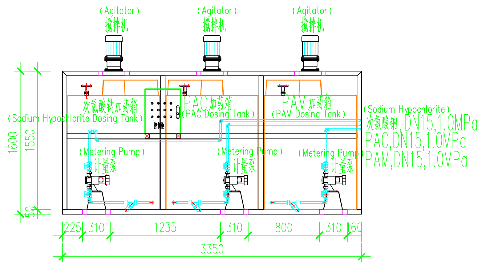
正视图 (Front View)
