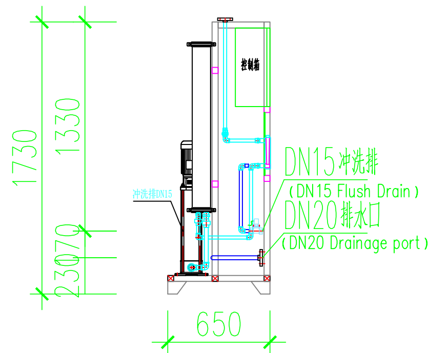
左视图 (Left View)
