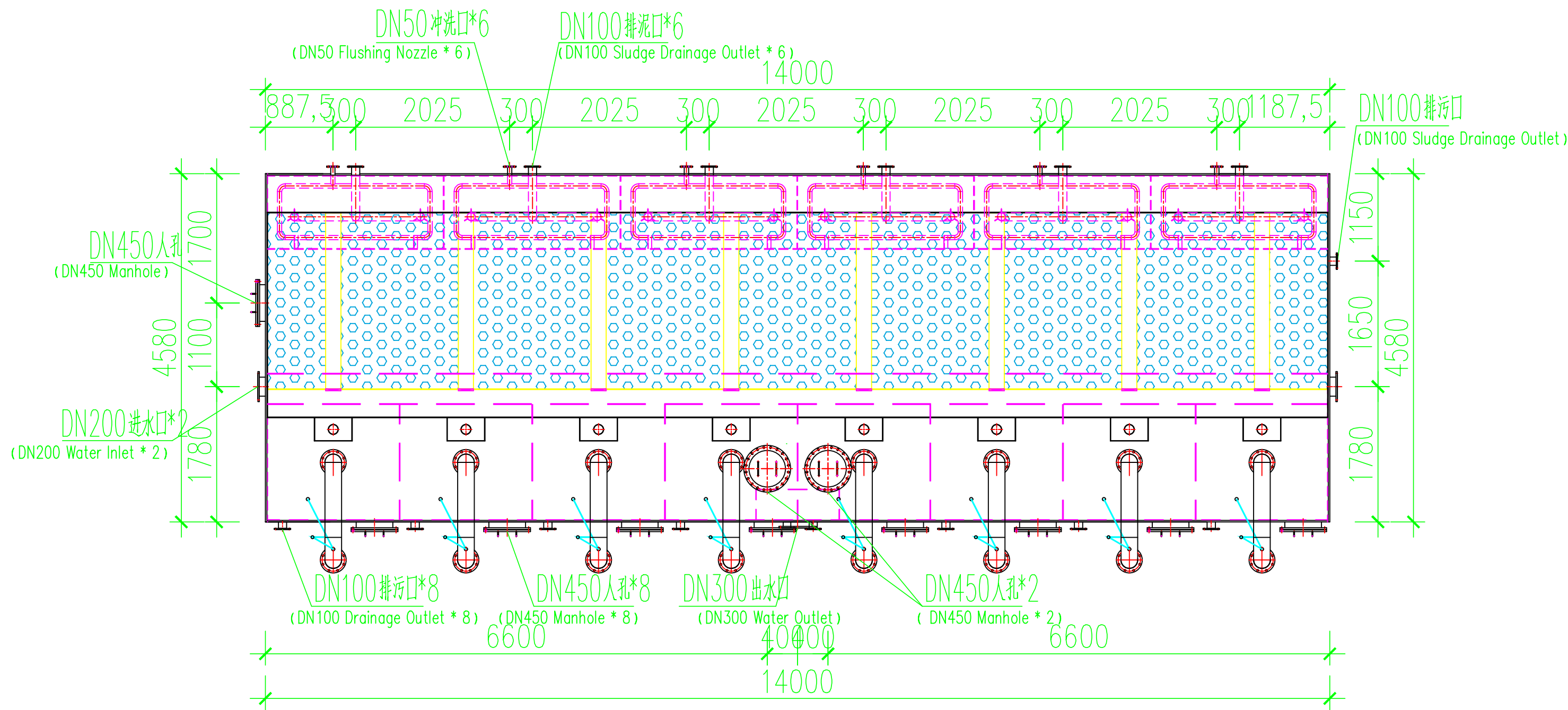
俯视图 (Top View)
