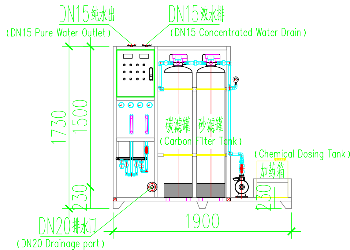
主视图 (Front View)
