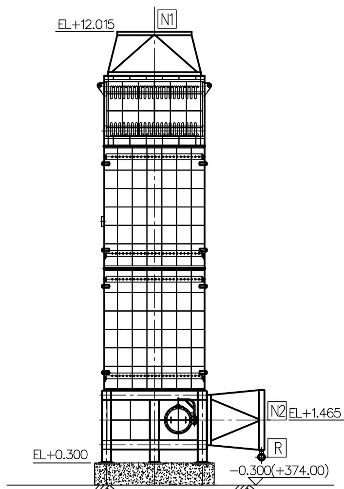
EX-11207 省煤器 4A Углесберегающий экономайзер 4A
