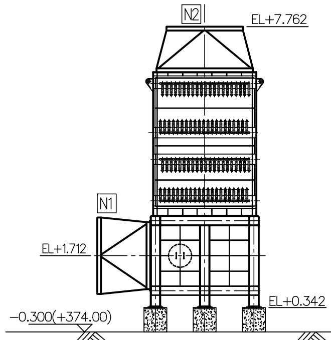
EX-11202 过热蒸汽 Пароперегреватель 1B
