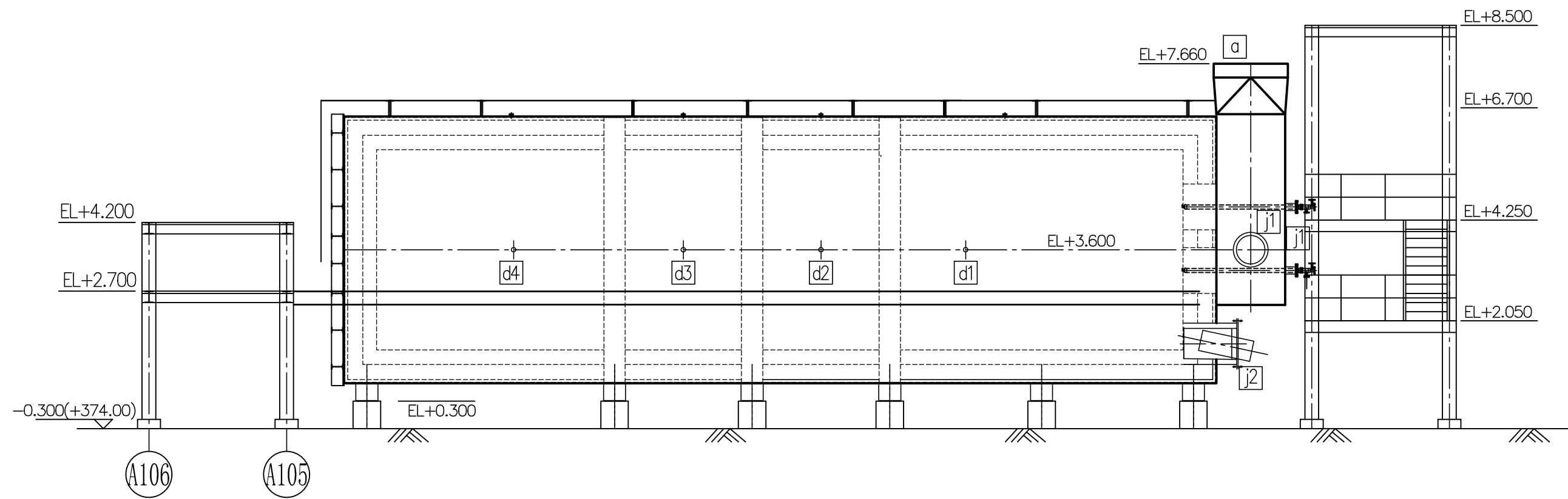
FU-11201 焚硫炉 Печь для сжигания серы
