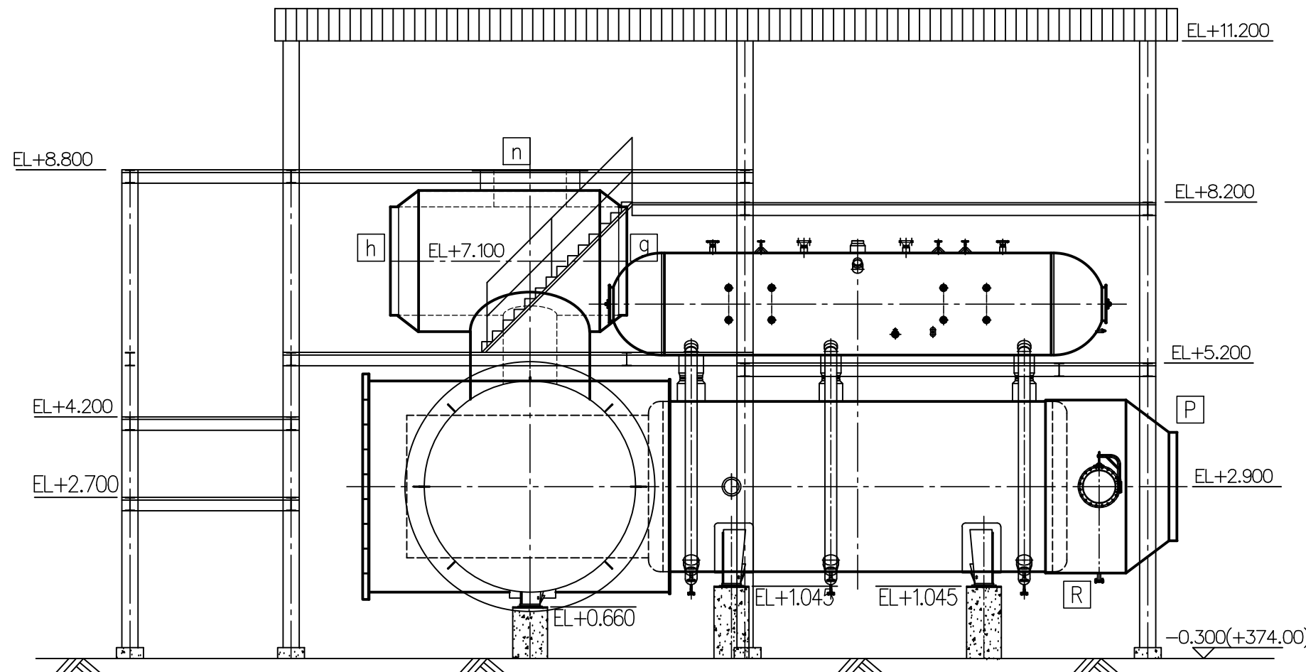
EX-11201 废热锅炉 Утилизационный котёл
