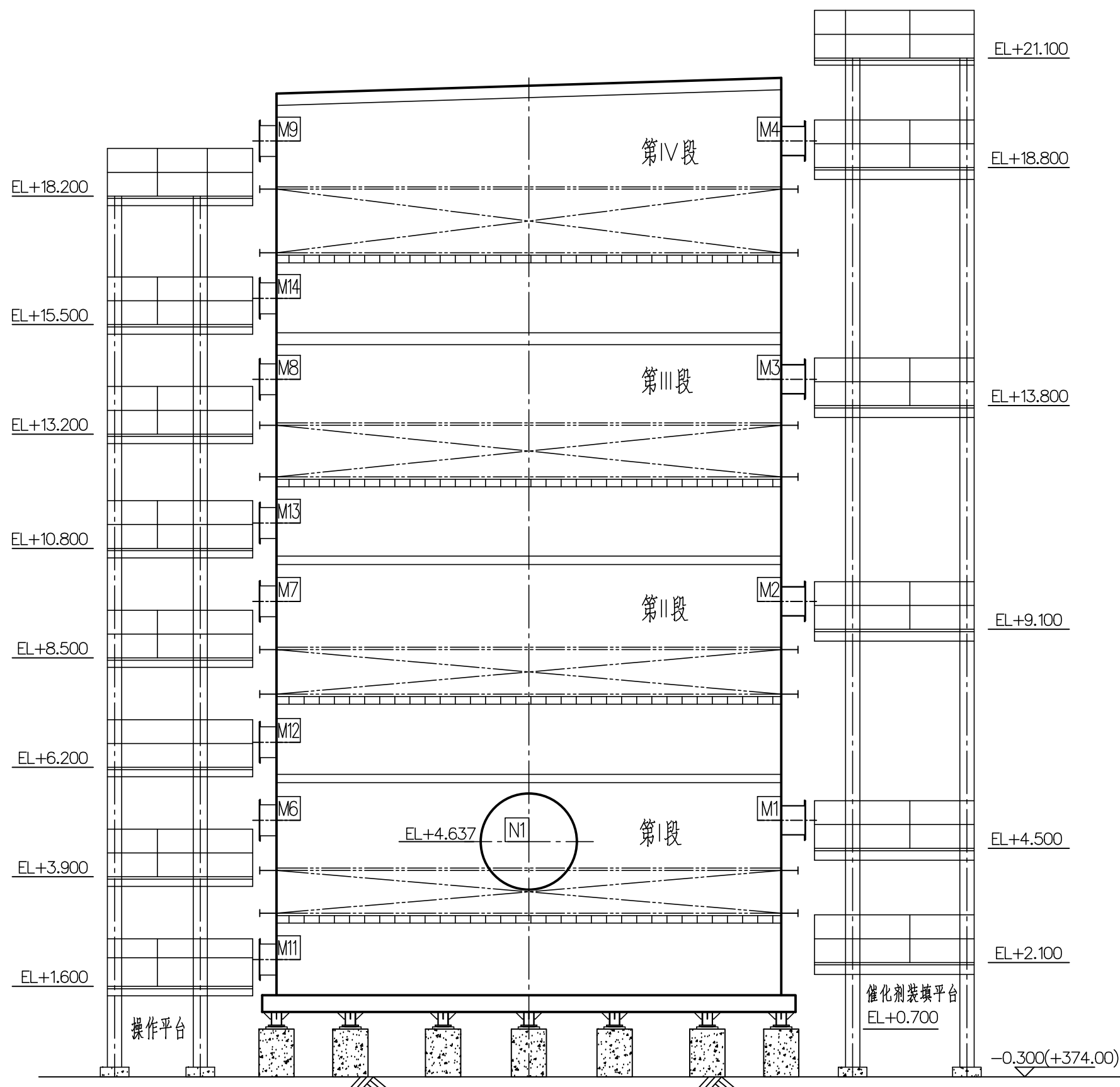
RE-11201 转化器 Конвертер
