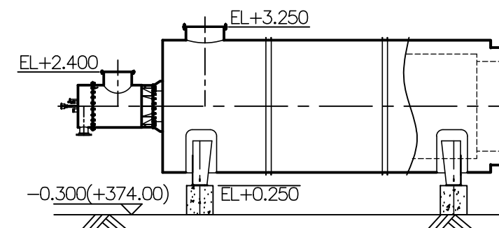
EX-11208 空气预热器 Воздухоподогреватель
