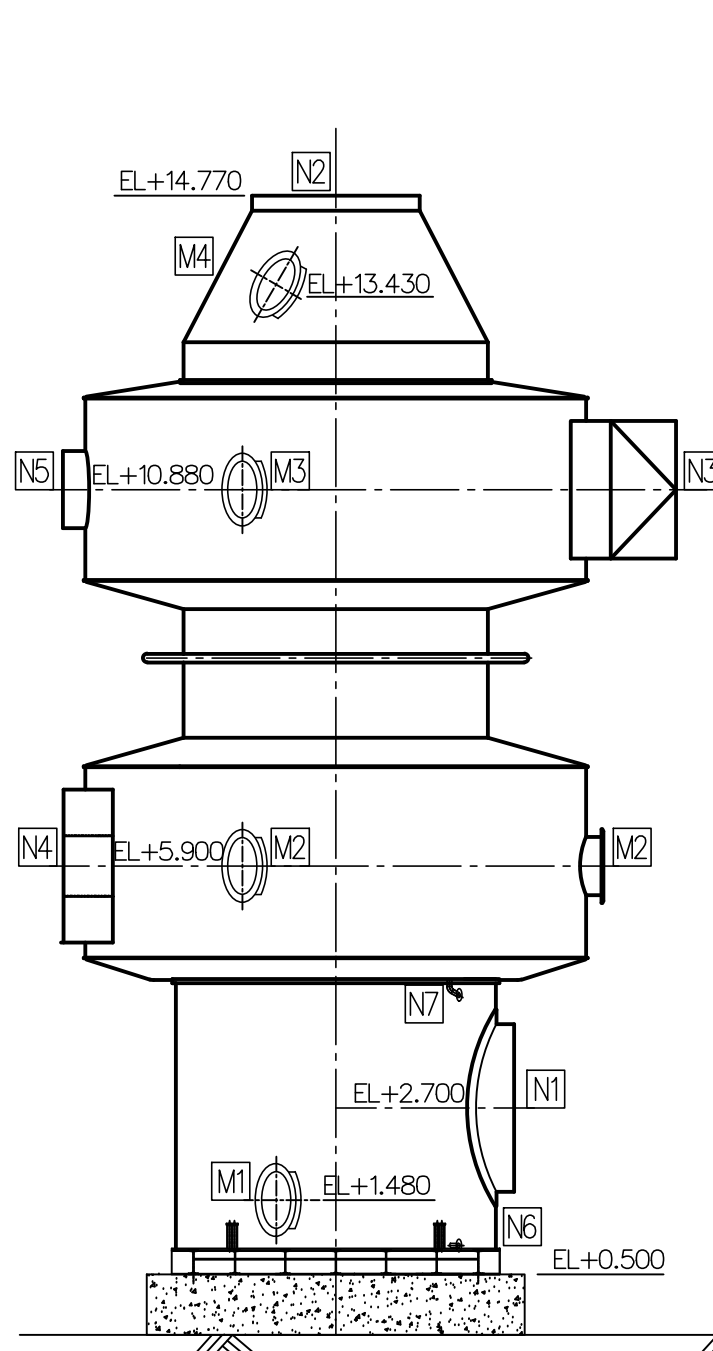
EX-11303 热交换器 Теплообменник холодных и горячих сред
