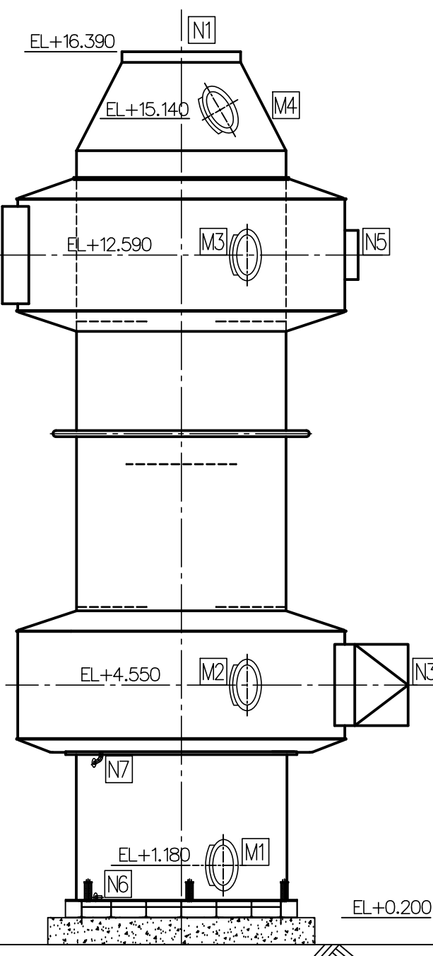
EX-11304 冷热交换器 Теплообменник холодных и горячих сред
