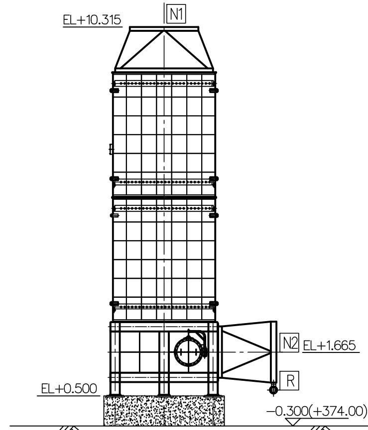
EX-11205 省煤器 3A Углесберегающий экономайзер 3A
