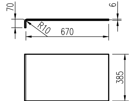
件号2详图 Детальный чертёж № 2 Не по соотношению 不按比例
