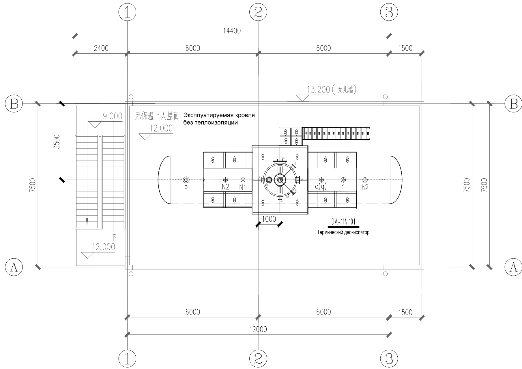
屋顶层设备布置平面图 1:100
