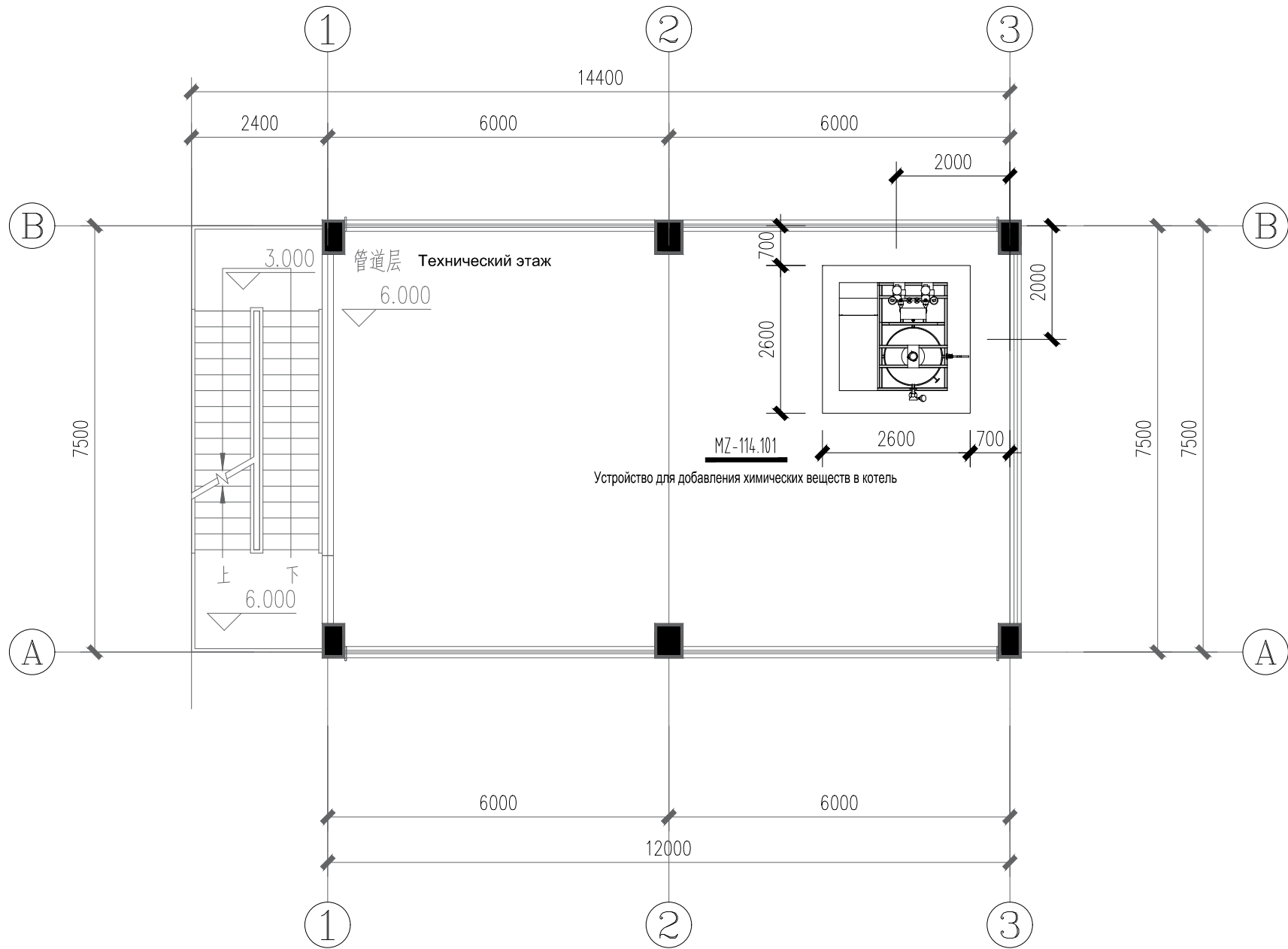
二层设备布置平面图 1:100
