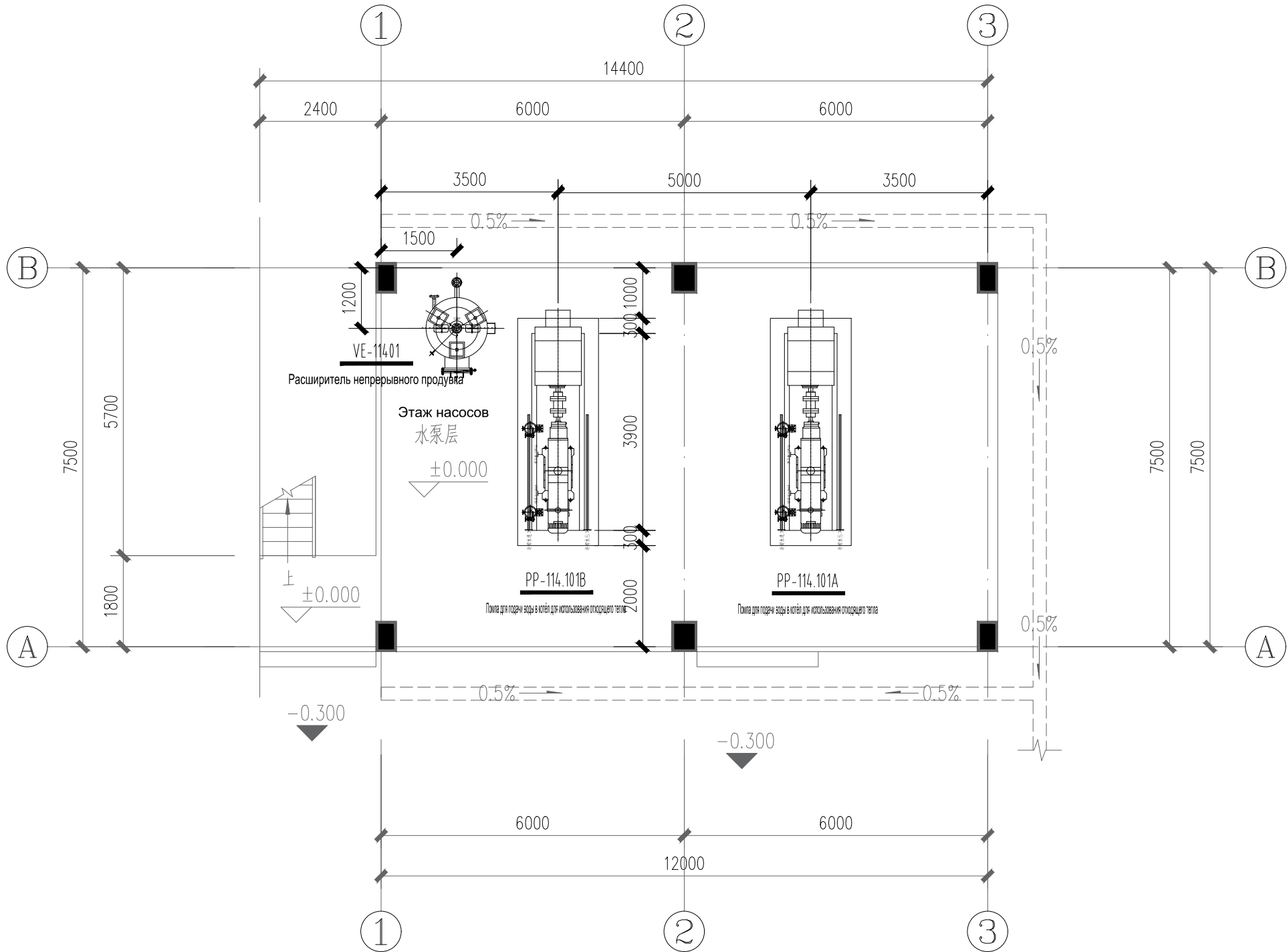
一层设备布置平面图 1:100
