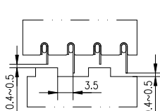
隔板汽封详图(C2、P1-P15) Detail of diaphragm gland
