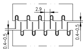
前汽封1段详图 Detail of front gland
