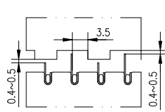
前汽封2、3、4段详图 Detail of front gland
