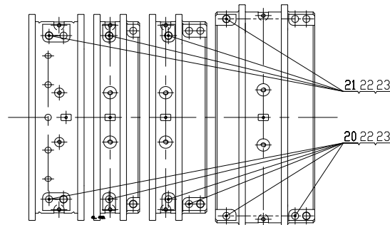
汽封详图 Details of gland
