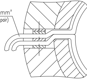
schematic lead-out wire for thermistor 热电阻引线引出示意图 A向
