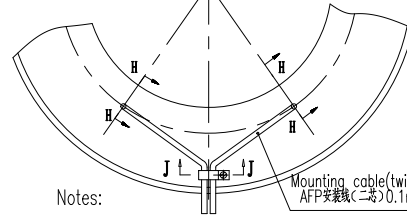
schematic lead-out wire for thermistor 热电阻引线引出示意图 A向
