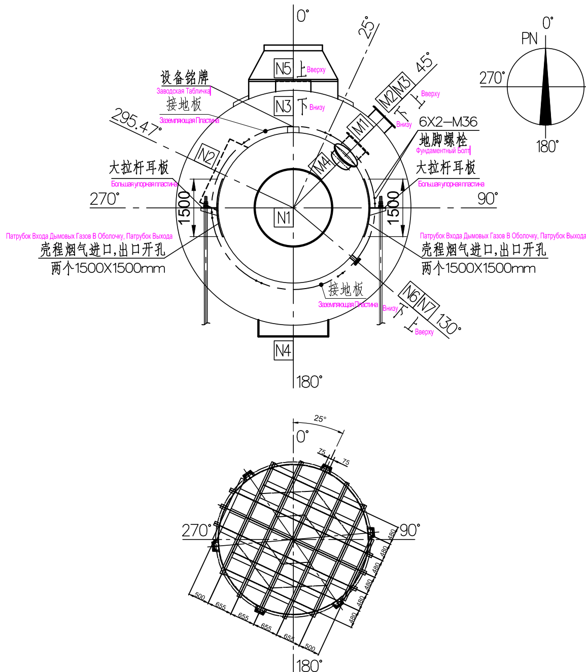
基础地脚螺栓与工字钢架布置图
