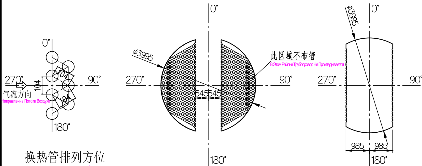
双弓折流板方位
