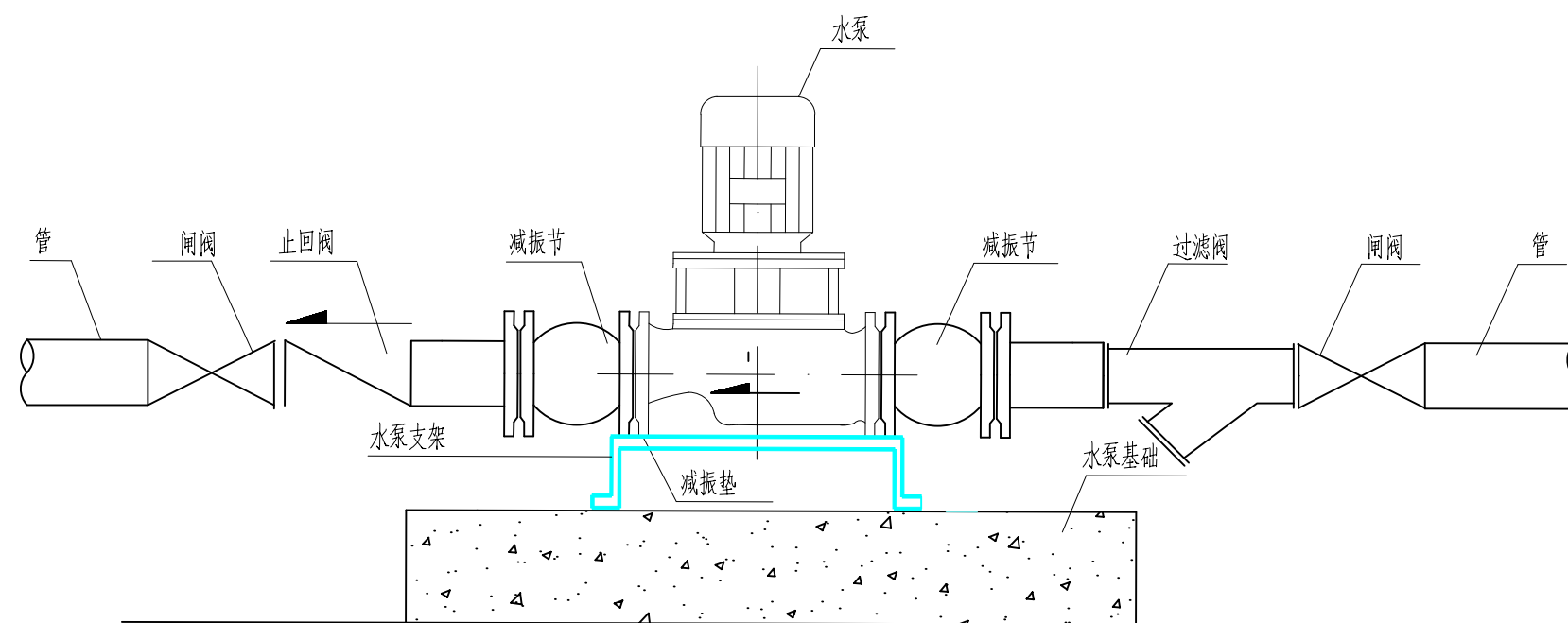
水泵安装大样图
