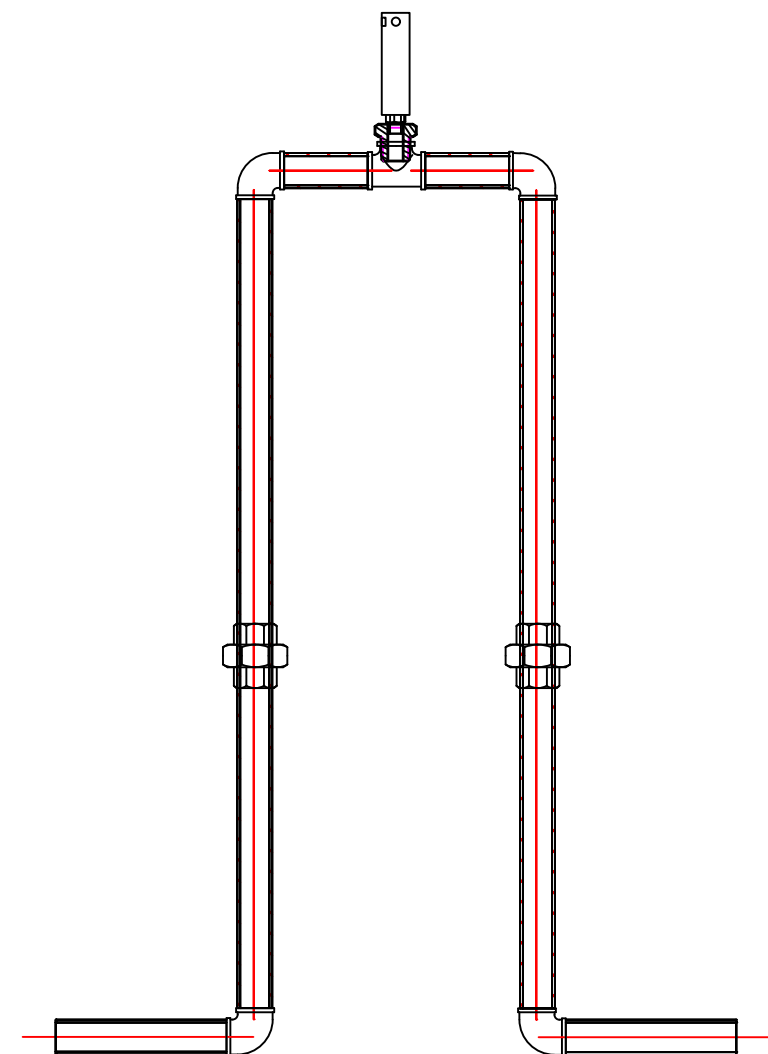
等高管安装大样图
