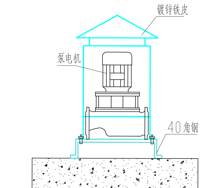
水泵防雨罩示意图
