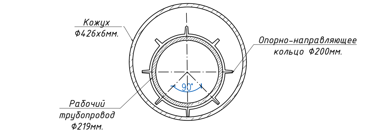
Футляр Сечение
