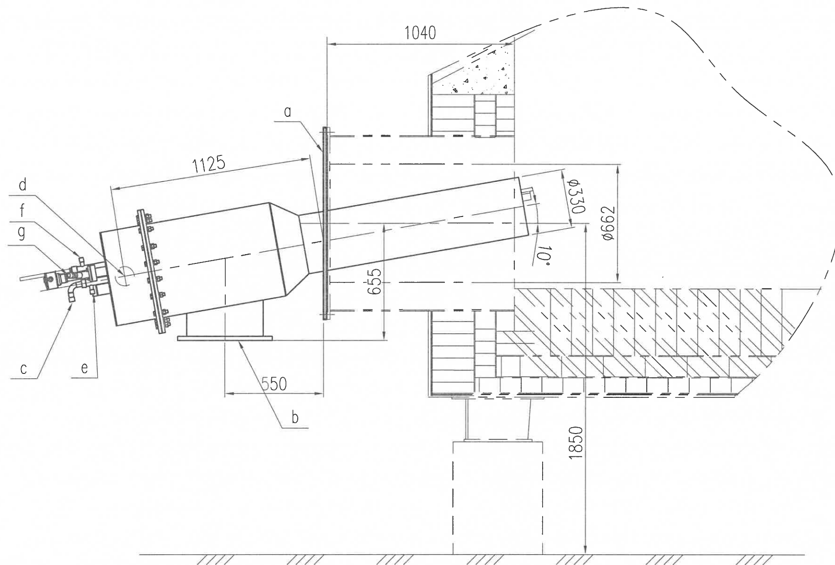
燃烧器安装尺寸配合图
