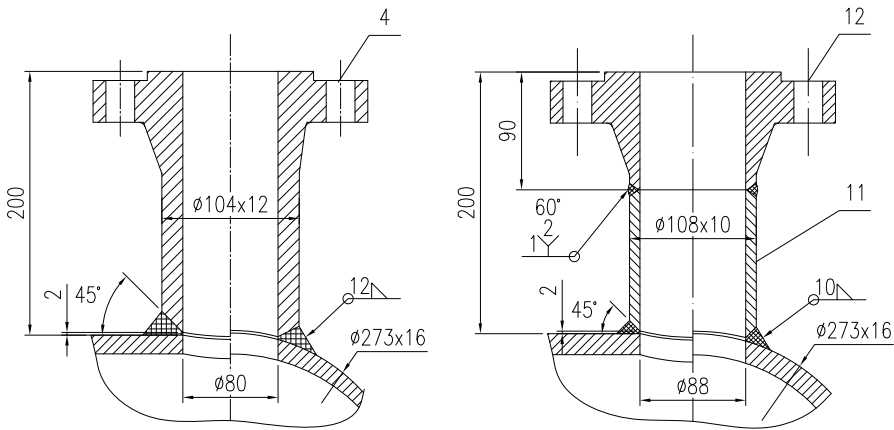
D接管(旋转) NOZZLE D DETAILSD (ROTATION) 1:2
