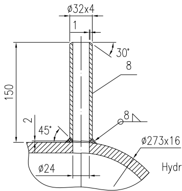
D接管(旋转) NOZZLE D DETAILSD (ROTATION) 1:2
