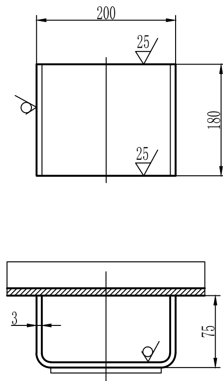
设备铭牌座 Основание таблички с техническими данными 不按比例 Без соблюдения масштаба
