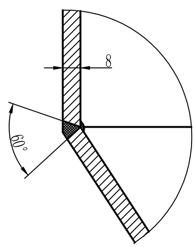
II II 不按比例 Без соблюдения масштаба
