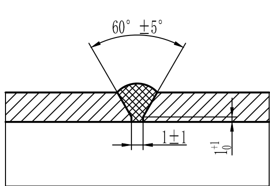
对接焊缝 Деталировка стыкового сварного шва 不按比例 Без соблюдения масштаба
