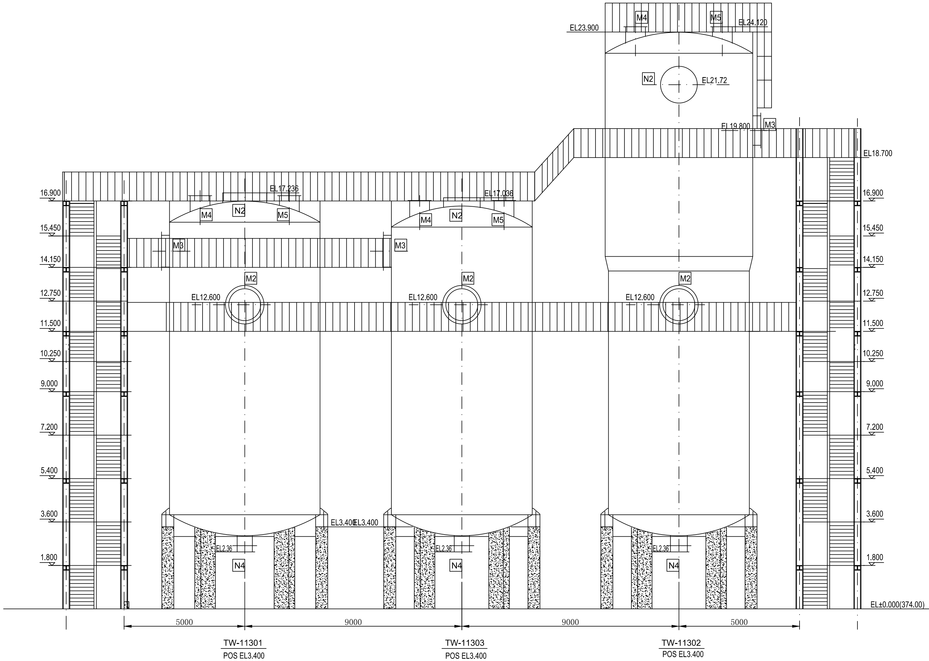
Разрез A-A A-A 剖面
