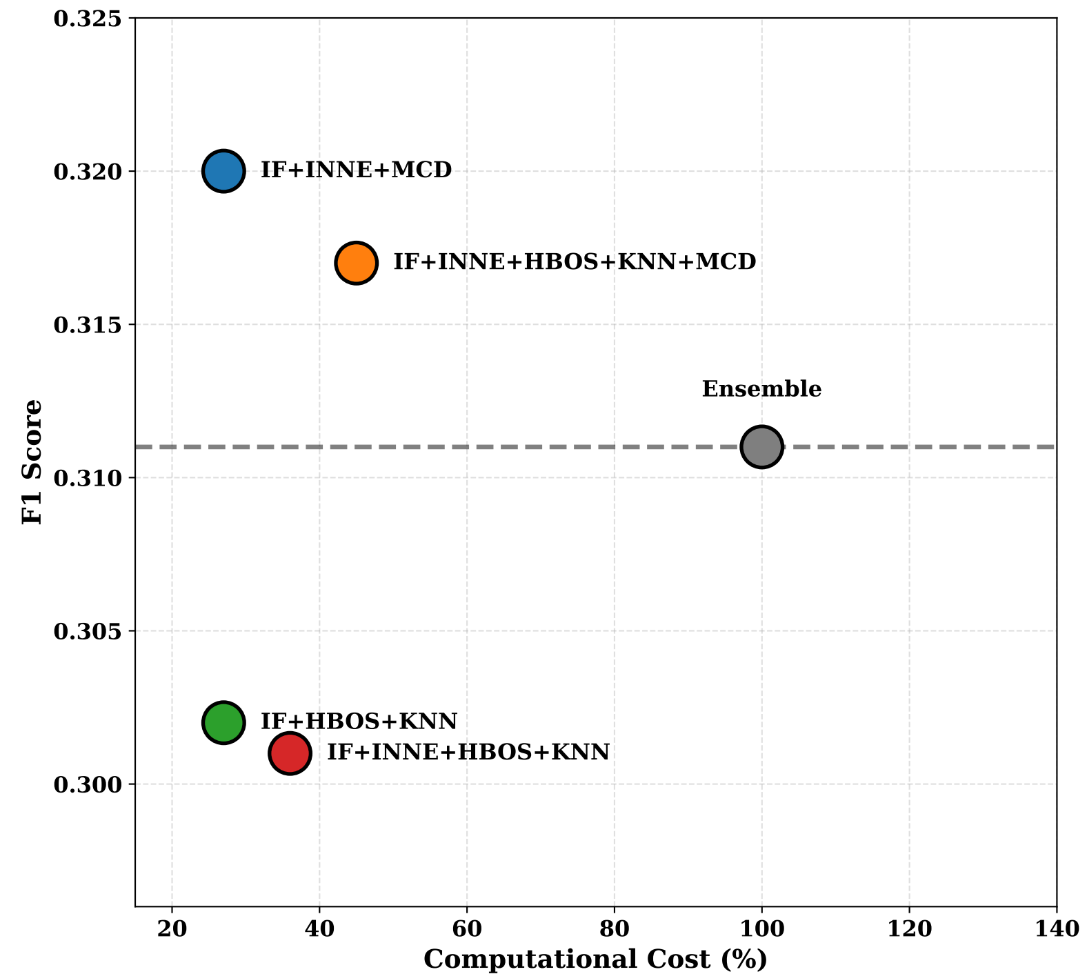
F1 Score vs Cost
