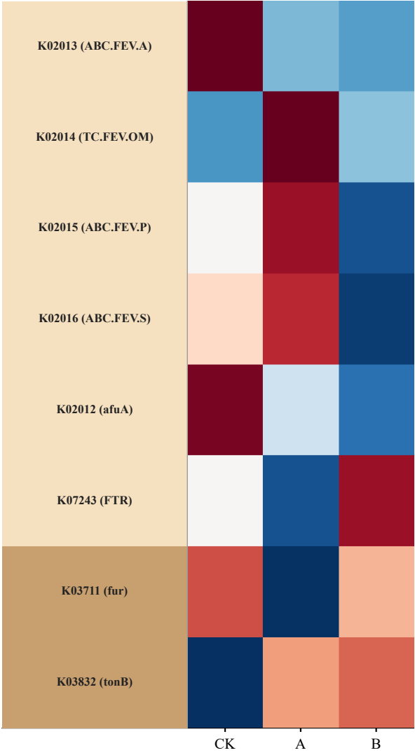
(d) 铁代谢
