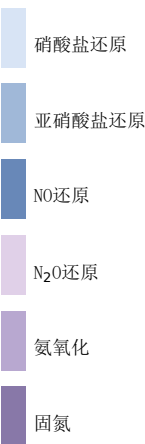
氮代谢
