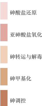
砷代谢
