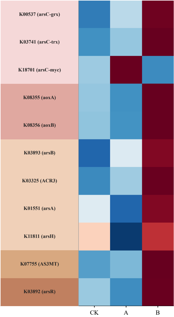
(a) 砷代谢
