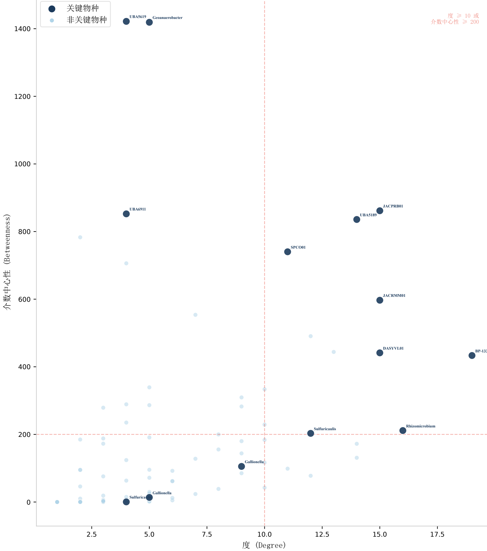
b. 关键物种筛选
