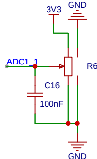
Potentiometer
