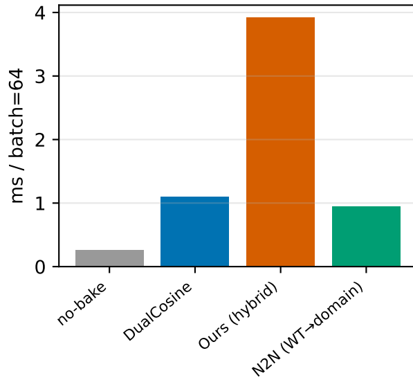
ptbxi ecg
