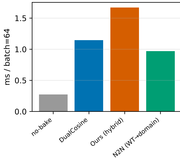
ptbxi ecg
