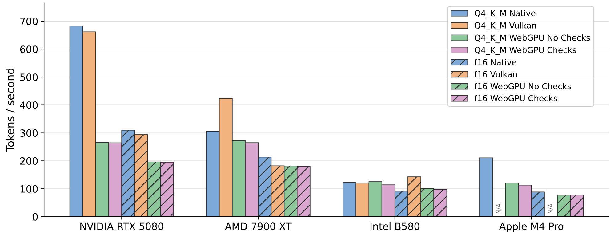
Llama 3.2 1B Decode Throughput
