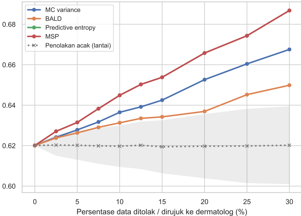
Akurasi vs Tingkat Rejeksi
