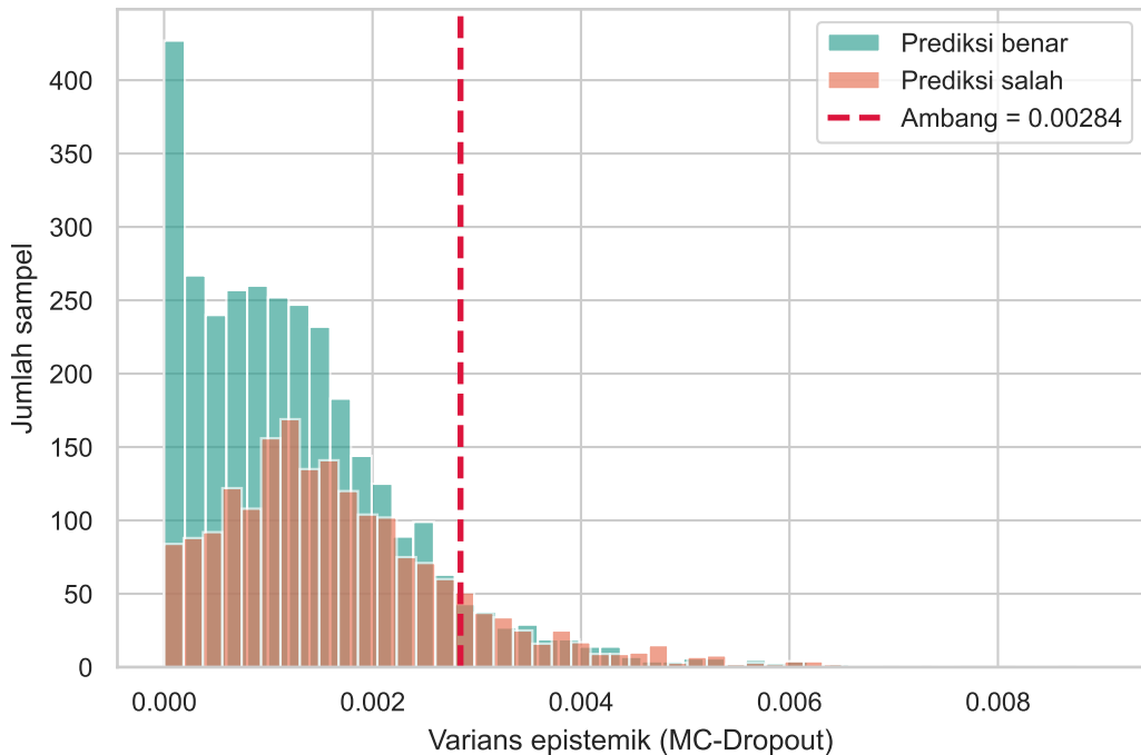
Distribusi ketidakpastian epistemik
