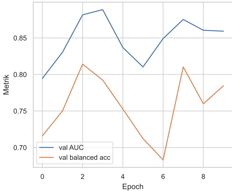
Stage 2 (oof) fold 0
