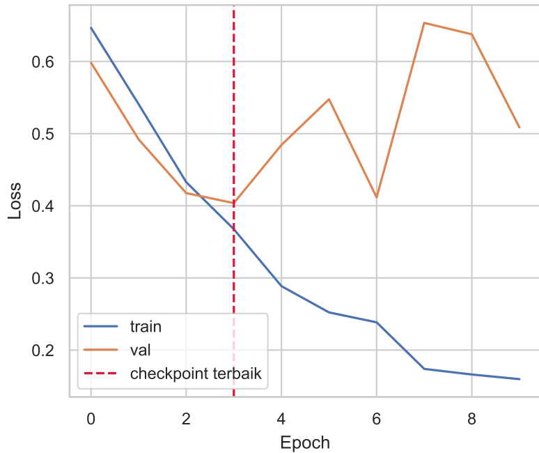
Stage 2 (oof) fold 1
