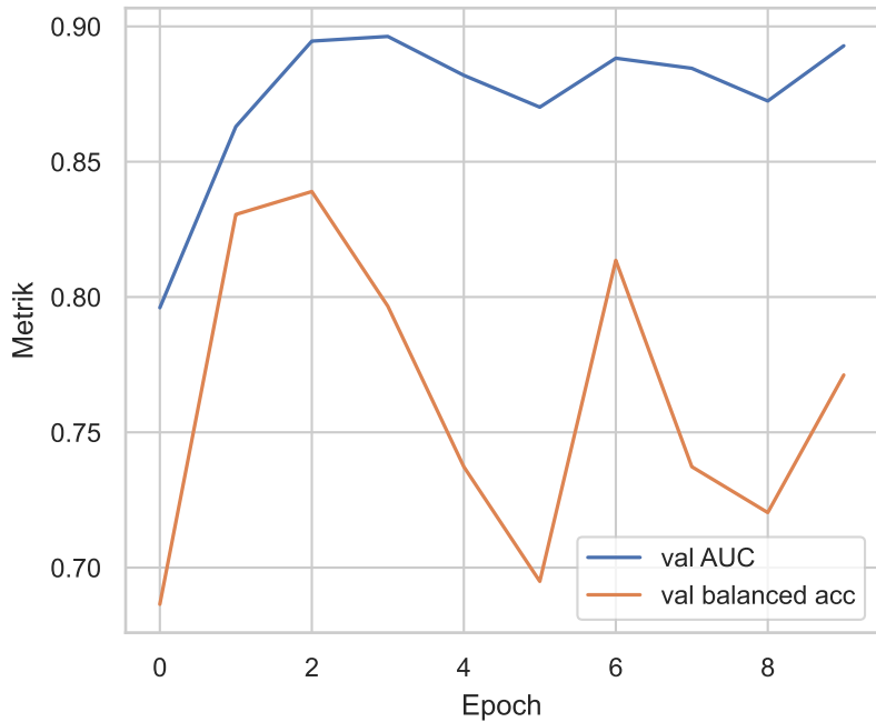
Stage 2 (oof) fold 1
