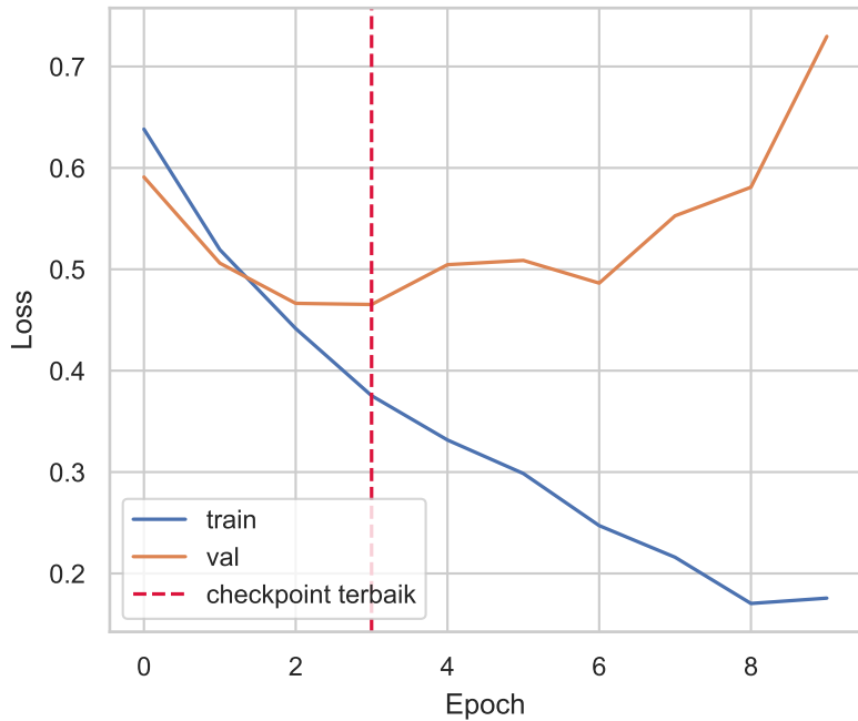
Stage 2 (oof) fold 2
