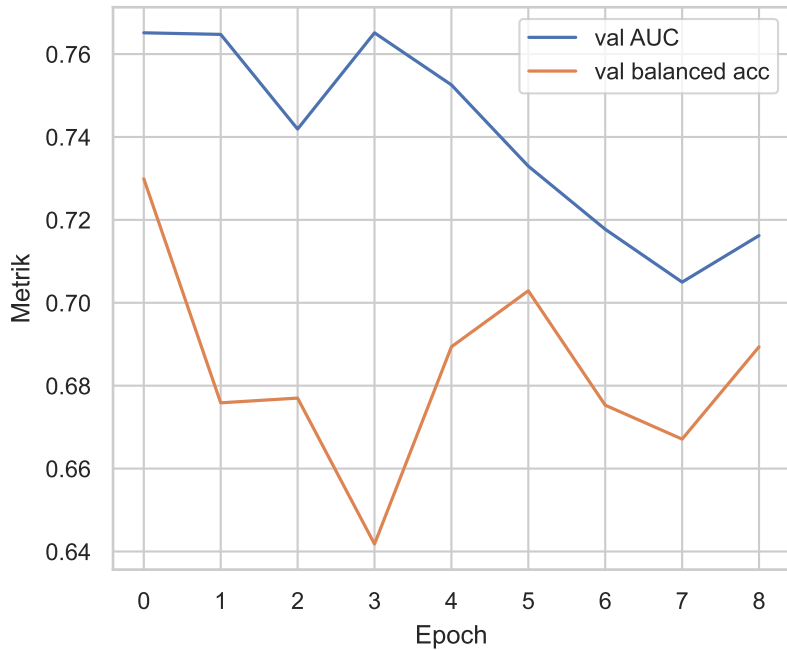
Stage 2 (oof) fold 4
