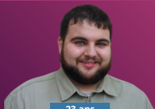
23 ans Nicolas GROS
