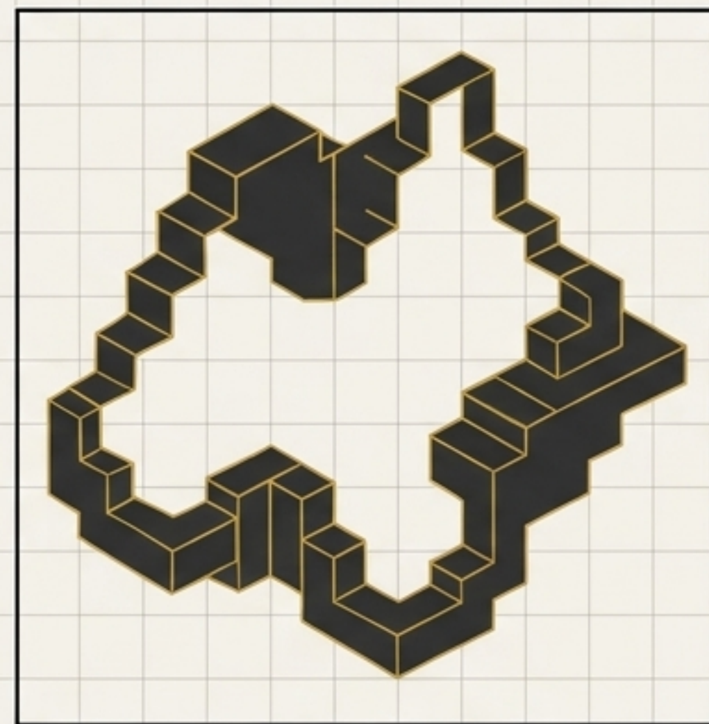
Exact-Integer Coordinates
